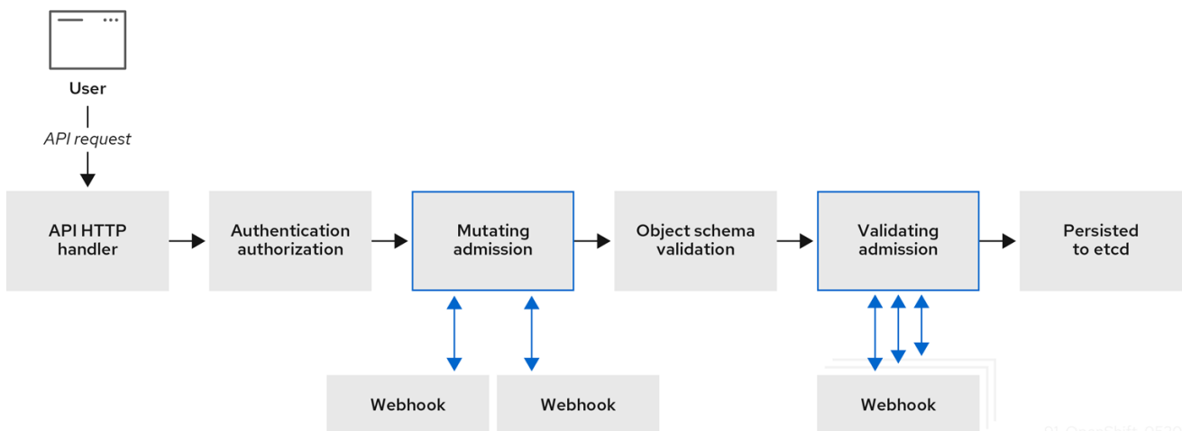
図9.1 変更用および検証用の受付プラグインを含む API 受付チェーン
