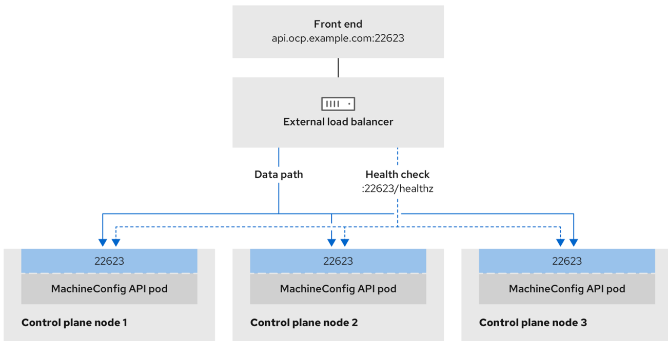
図24.3 OpenShift Container Platform 環境で動作する OpenShift MachineConfig API を示すネットワークワークフローの例
