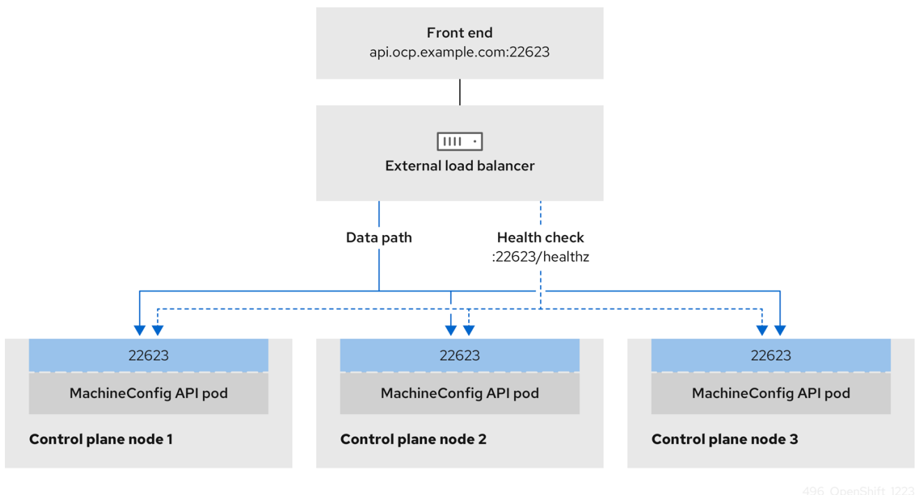
図24.12 OpenShift Container Platform 環境で動作する OpenShift MachineConfig API を示すネットワークワークフローの例
