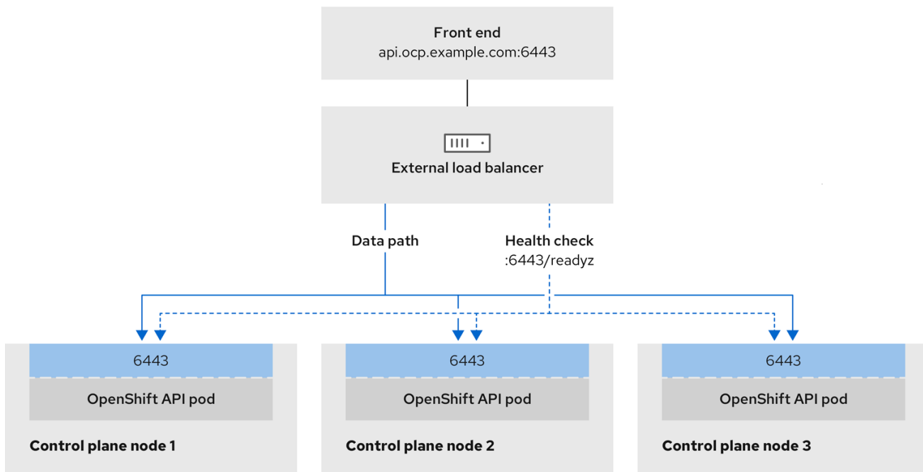
図24.2 OpenShift Container Platform 環境で動作する OpenShift API を示すネットワークワークフローの例
