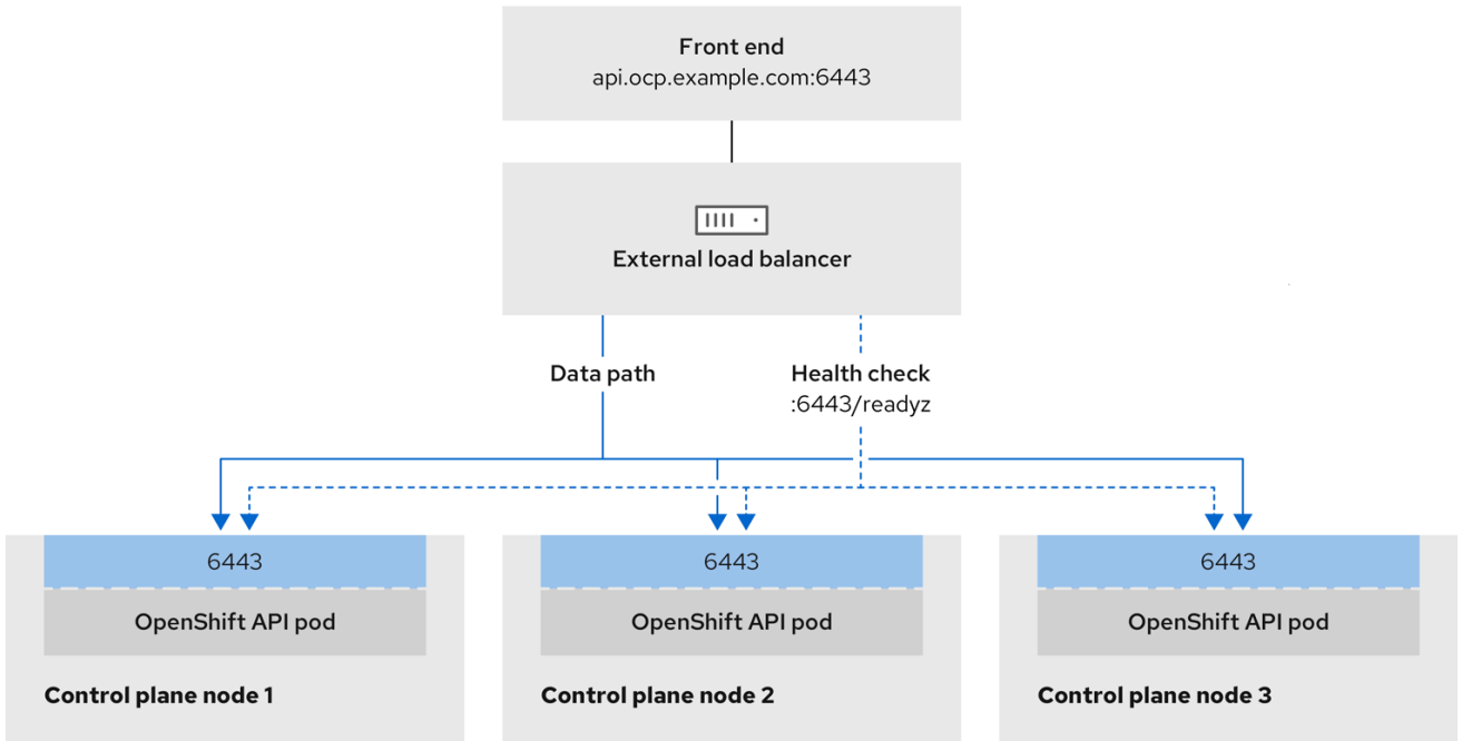
図23.2 OpenShift Container Platform 環境で動作する OpenShift API を示すネットワークワークフローの例
