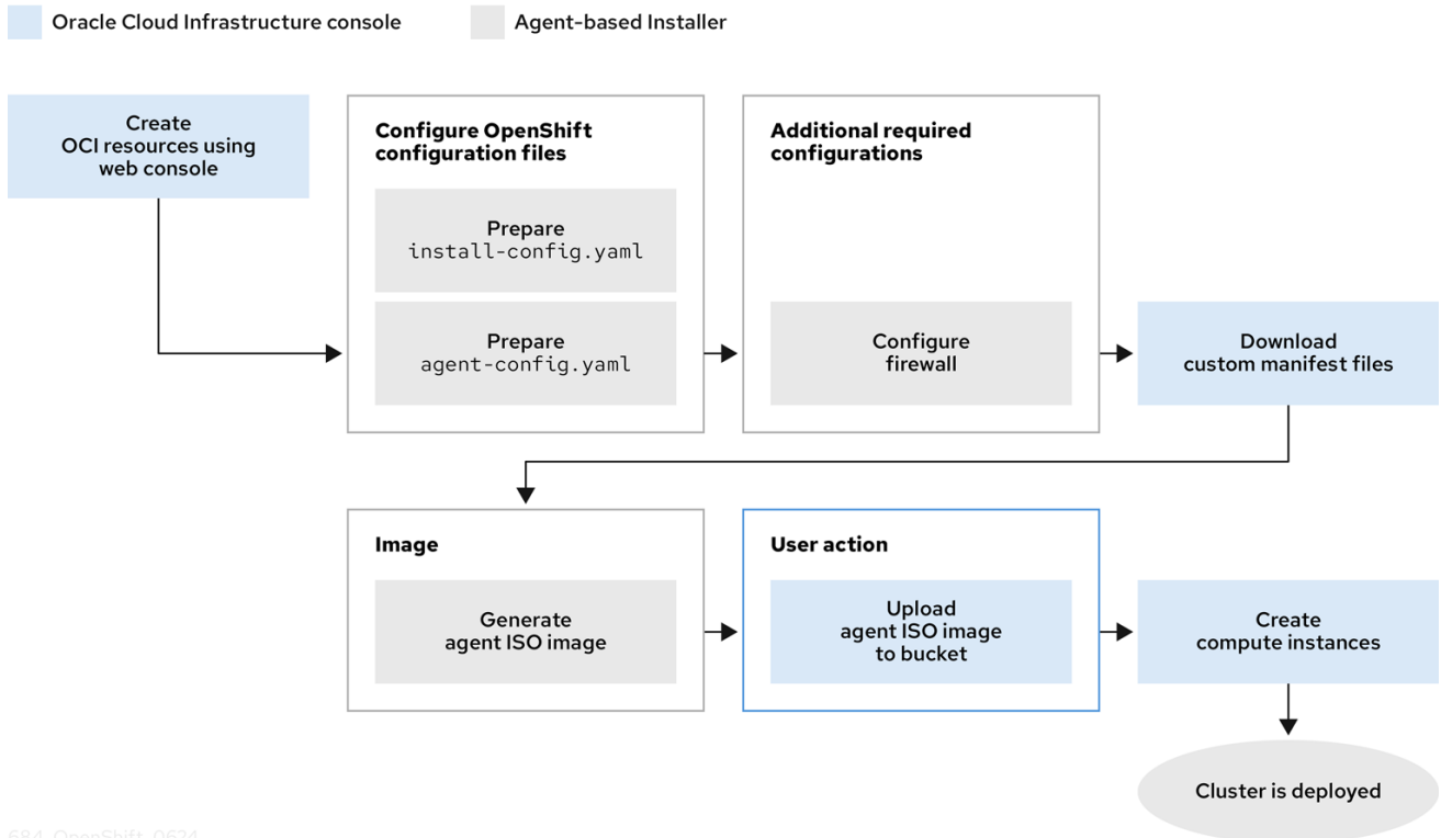
図22.2 接続環境でエージェントベースのインストーラーを使用して OCI にクラスターをインストールするためのワークフロー
