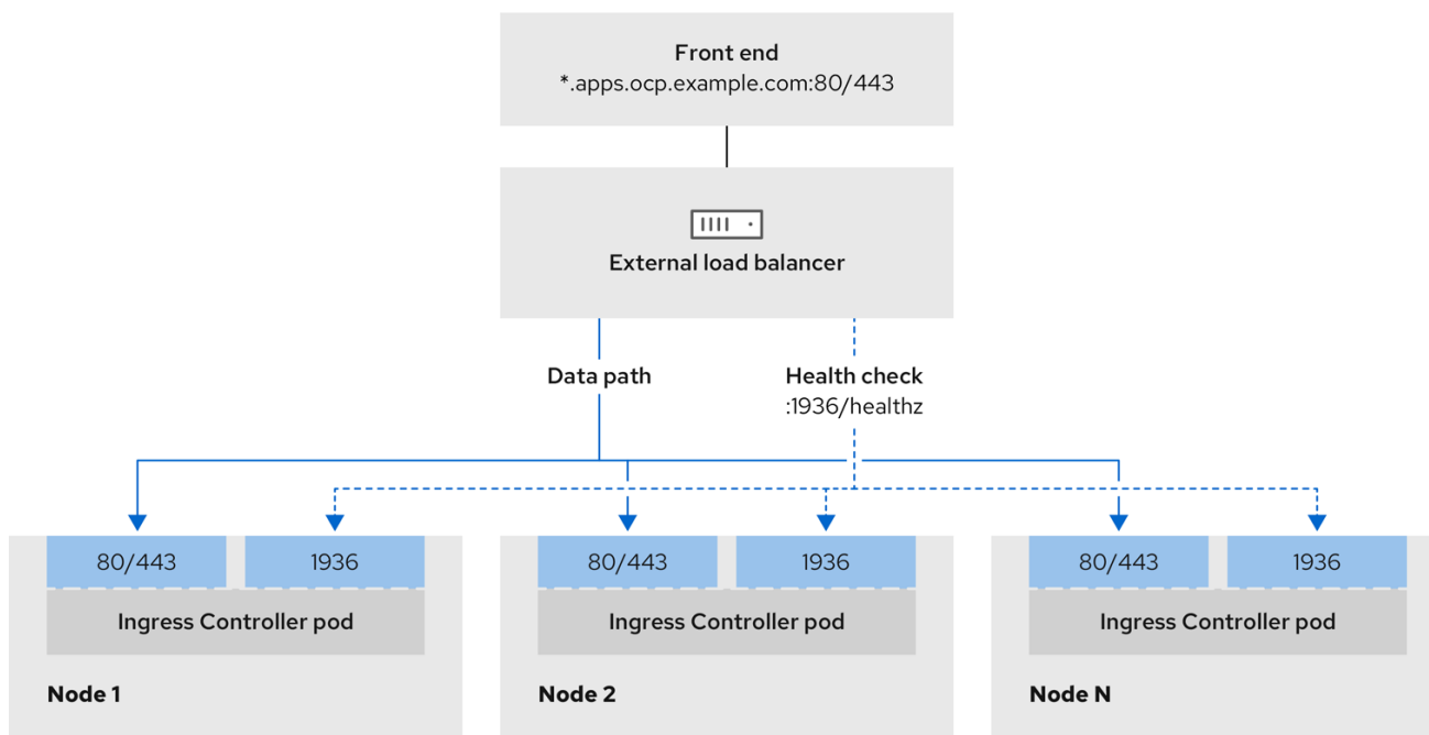
図23.7 OpenShift Container Platform 環境で動作する Ingress Controller を示すネットワークワークフローの例
