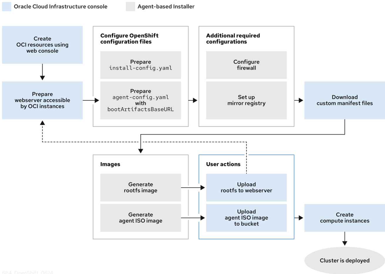
図22.3 切断された環境でエージェントベースのインストーラーを使用して OCI にクラスターをインストールするためのワークフロー
