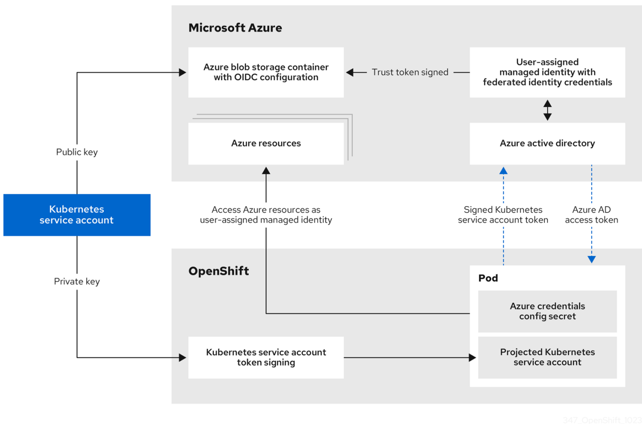
図19.4 ワークロード ID 認証フロー
