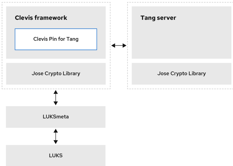
図17.1 LUKS1で暗号化したボリュームを使用する場合の NBDE スキーム(luksmeta パッケージは、LUKS2 ボリュームには使用されません)
