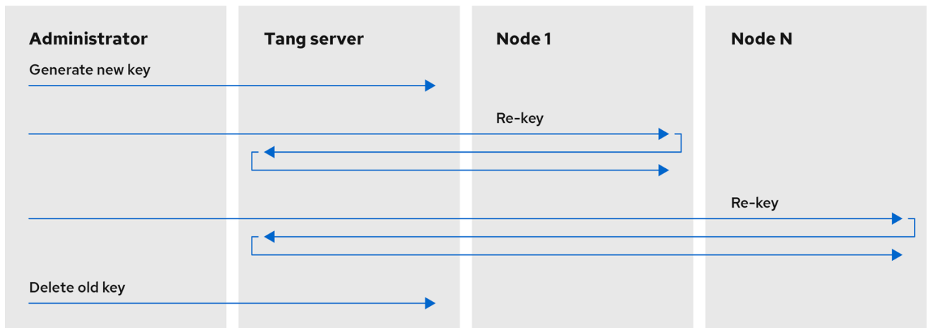
図17.2 Tang サーバーのキー再生成のワークフロー例
