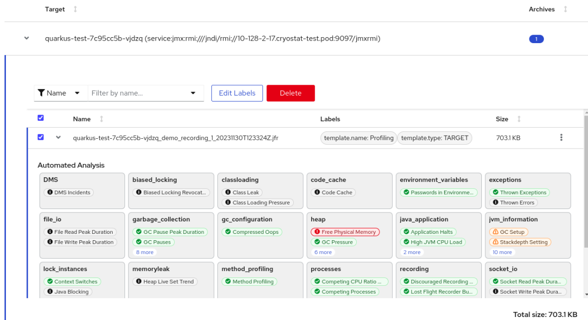
図2.3 アーカイブされた JFR レコーディングの削除
