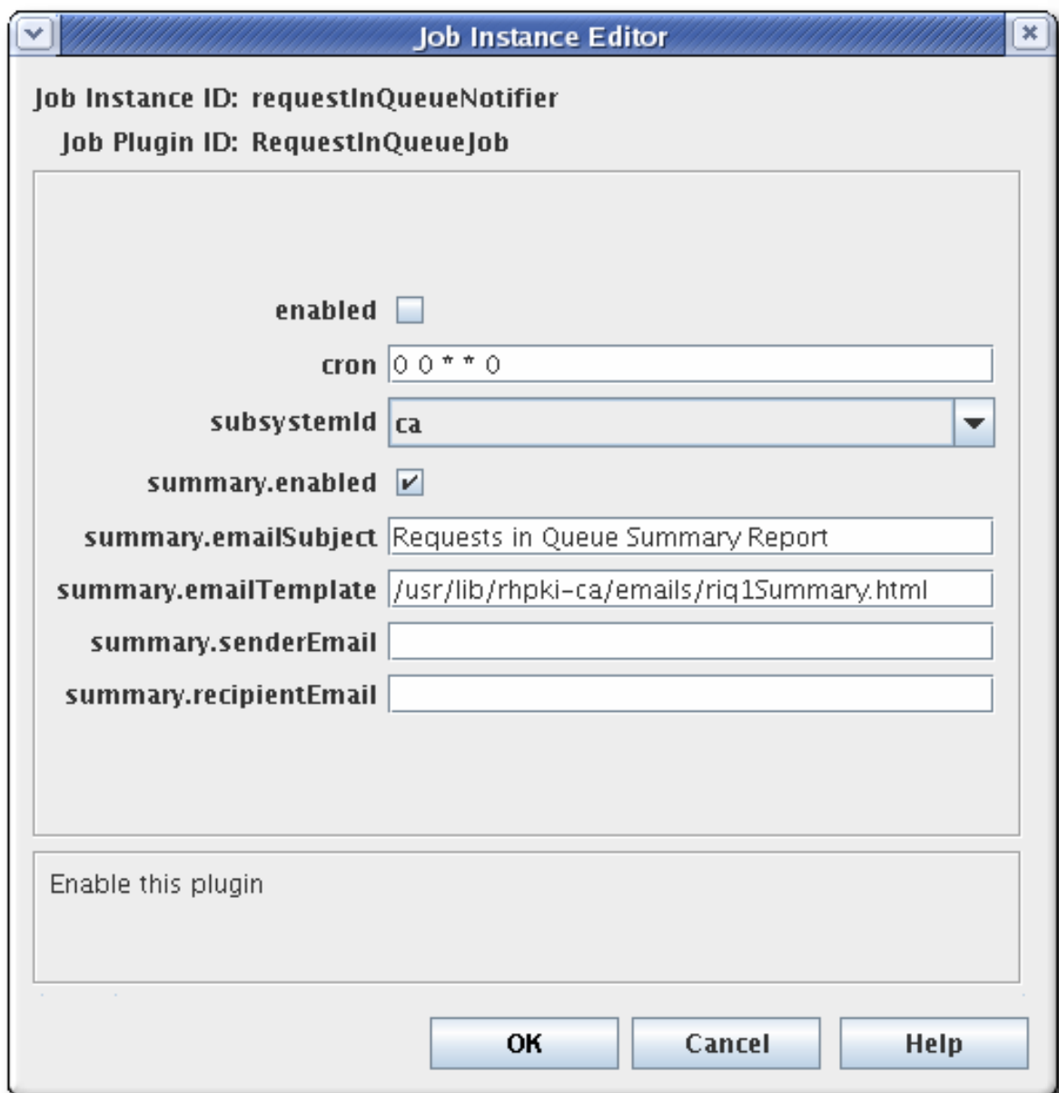
図12.1 ジョブ設定
