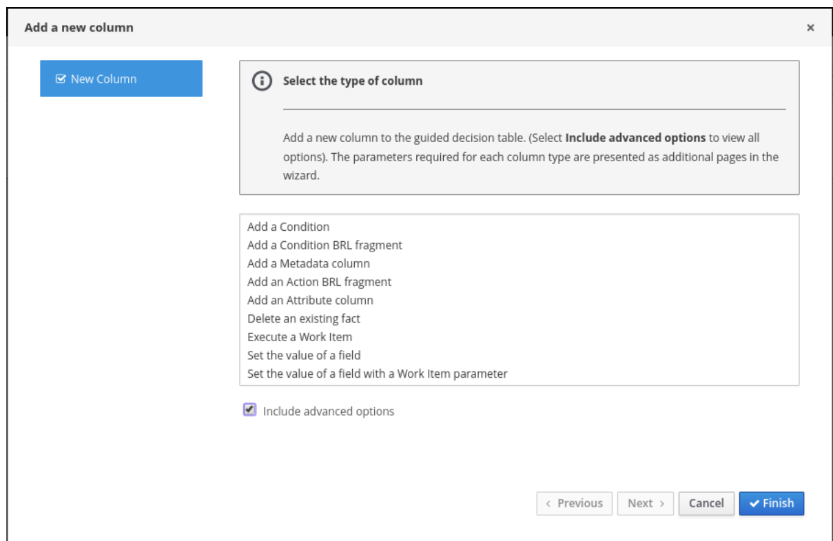
图6.1 Add columns
