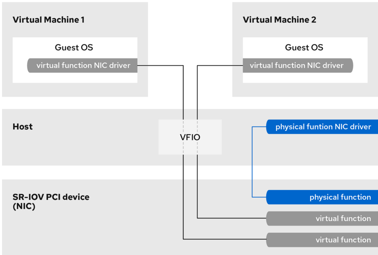
図11.1 SR-IOV アーキテクチャー
