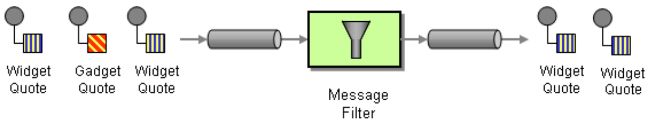
図8.2 Message Filter パターン
