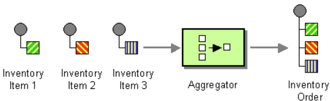
図8.5 Aggregator パターン
