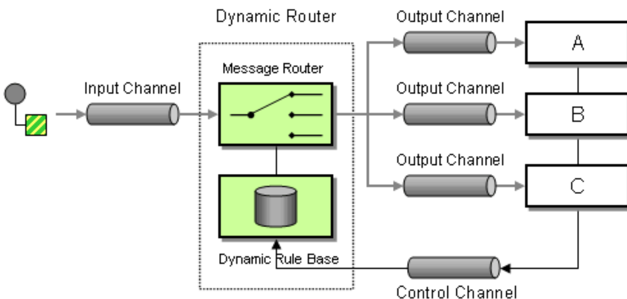
図8.12 Dynamic Router パターン
