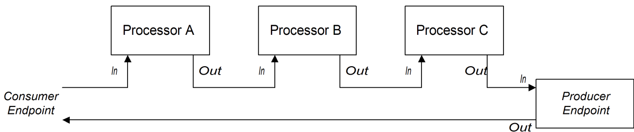
図2.4 InOut エクスチェンジのサンプルパイプライン
