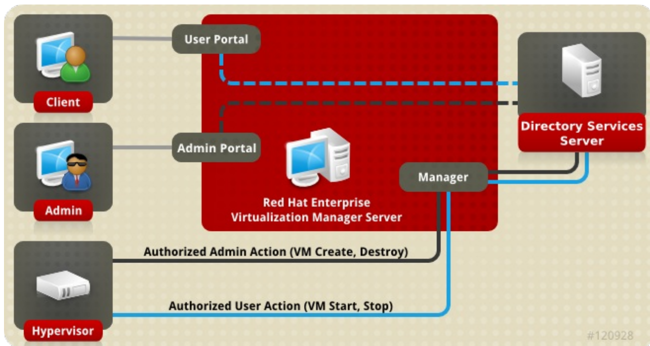
図6.1 GSSAPI 認証
