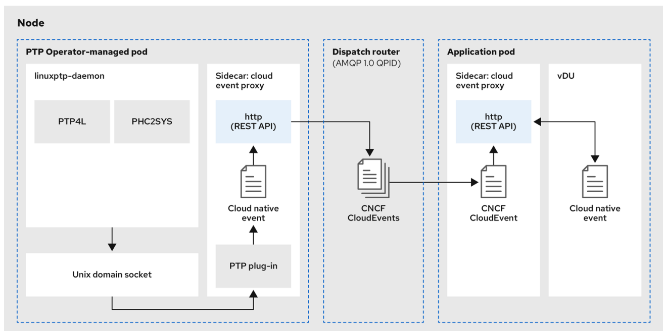
図15.1 PTP 高速イベントの概要
