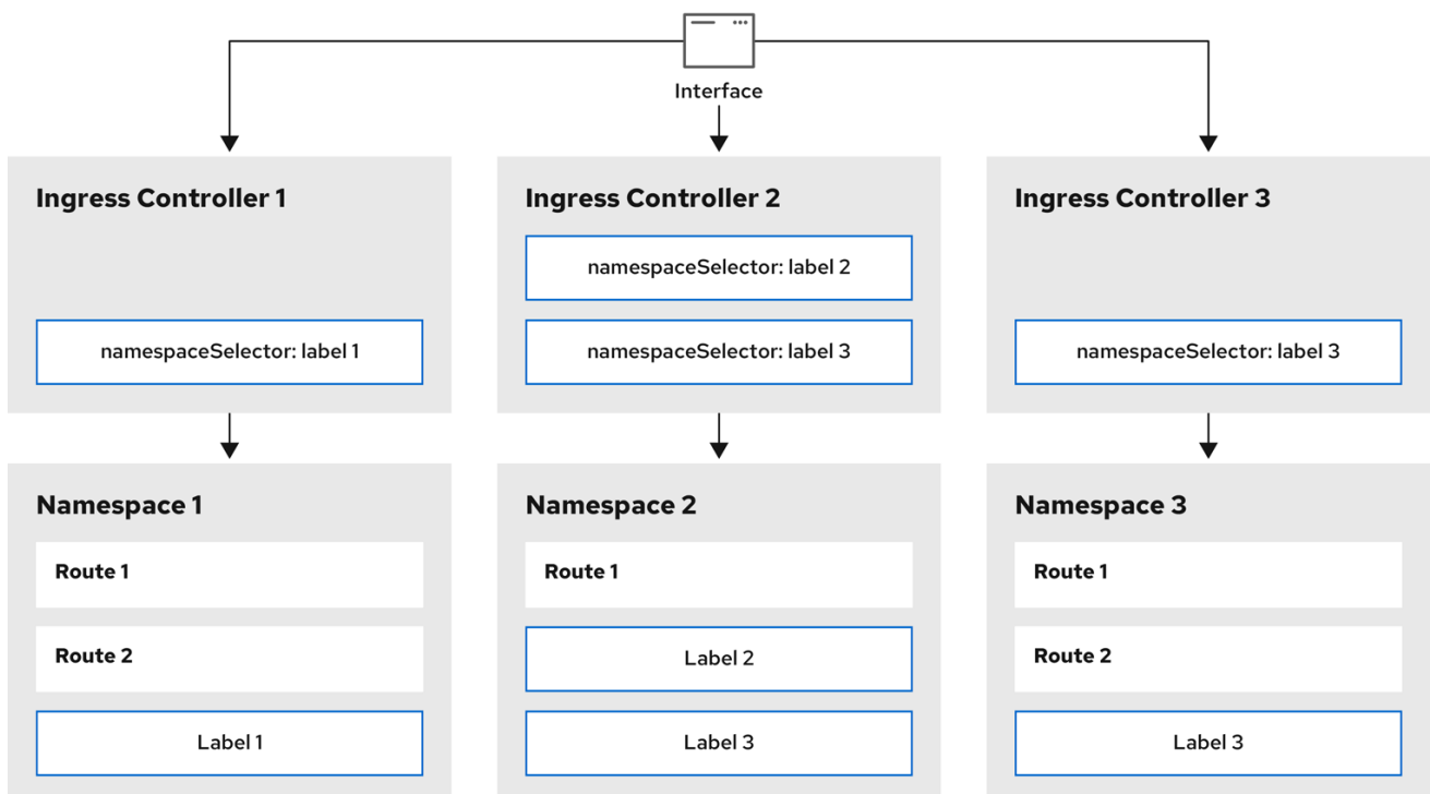
図25.2 namespace ラベルを使用した Ingress シャーディング
