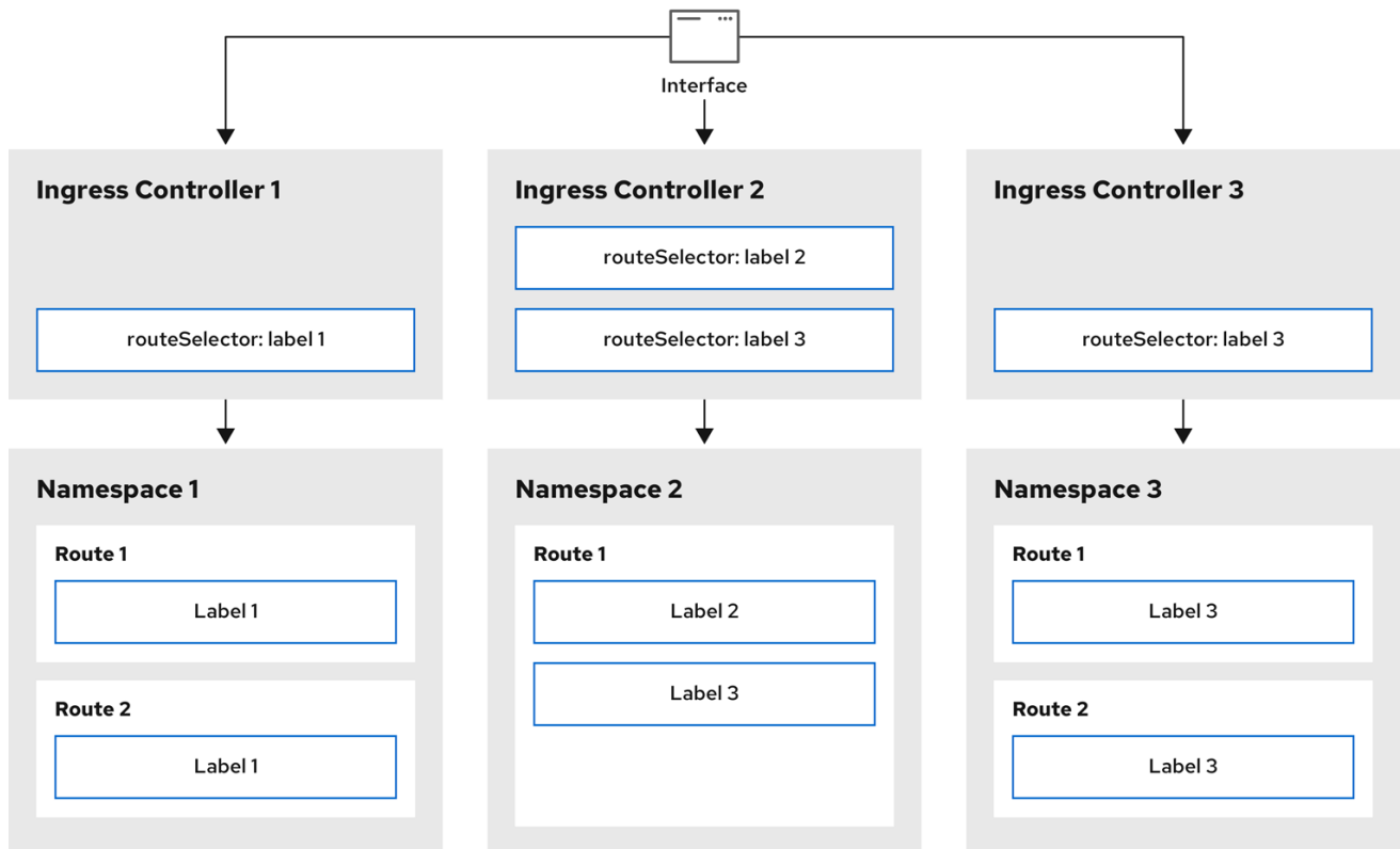
図25.1 ルートラベルを使用した Ingress シャーディング
