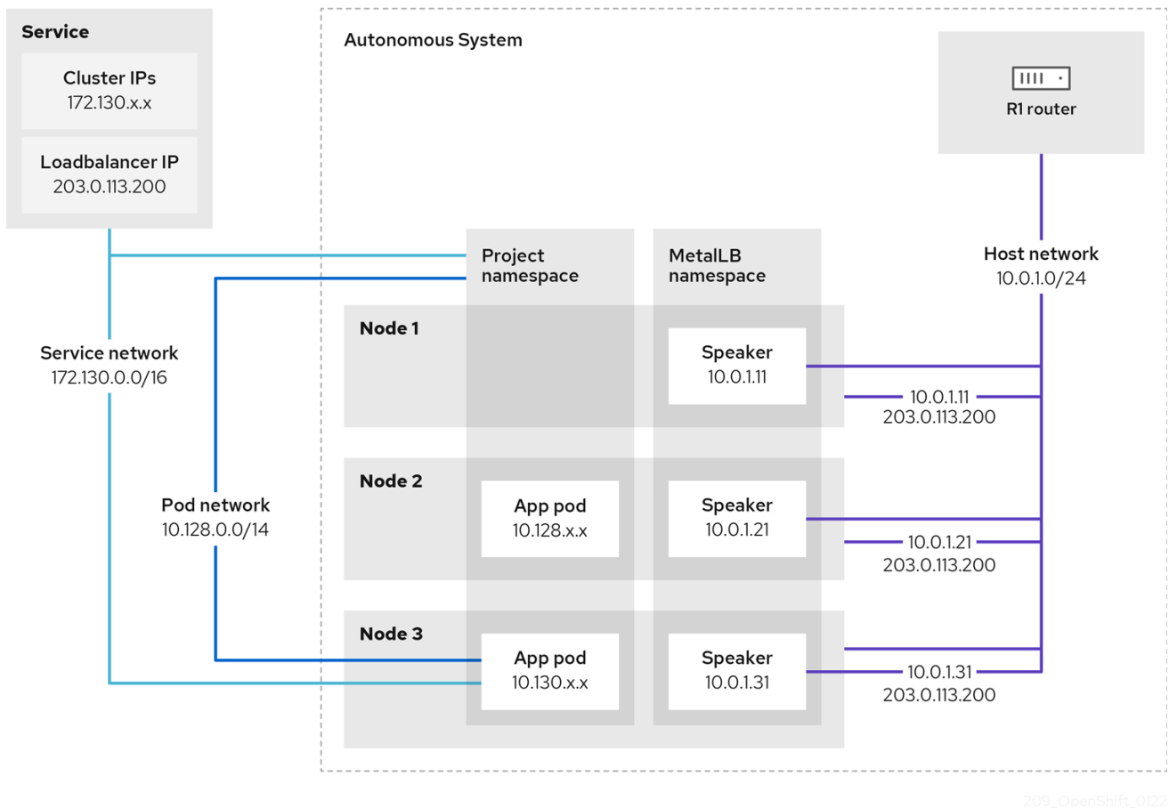
図30.1 BGP モードの MetalLB トポロジーの図
