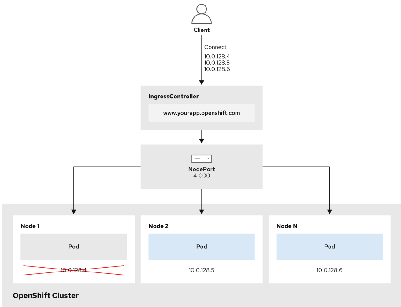
図8.1 NodePortService の図
