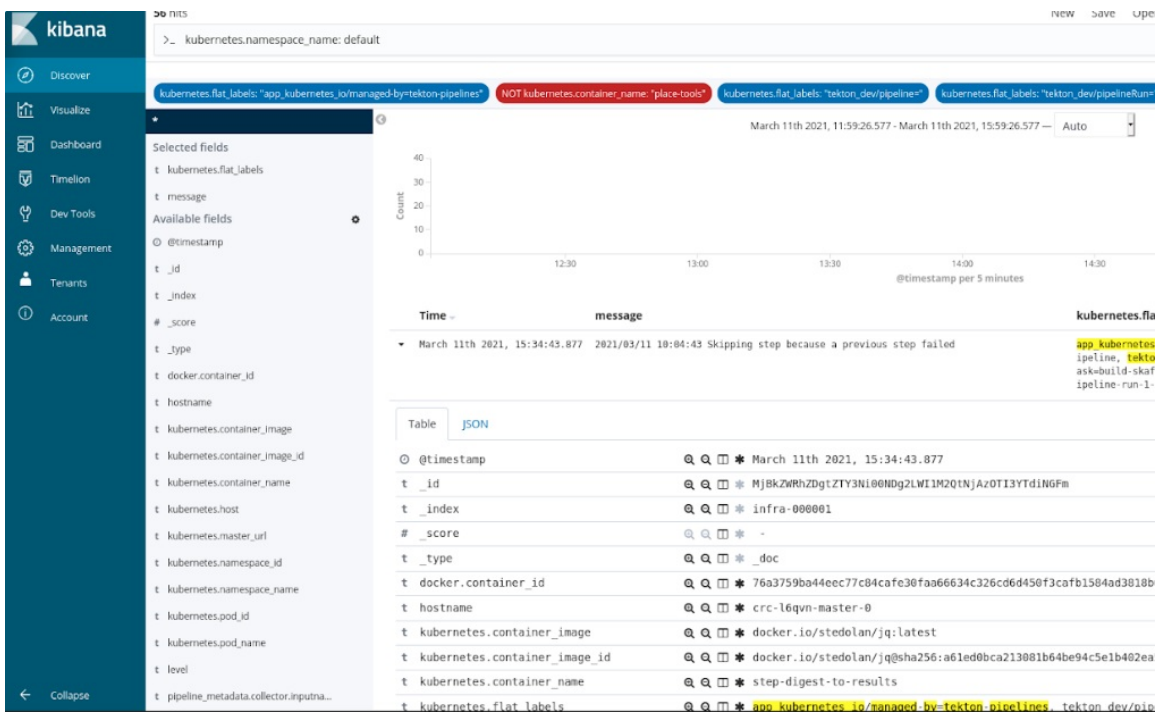
그림 3.7. 필터링된 메시지
