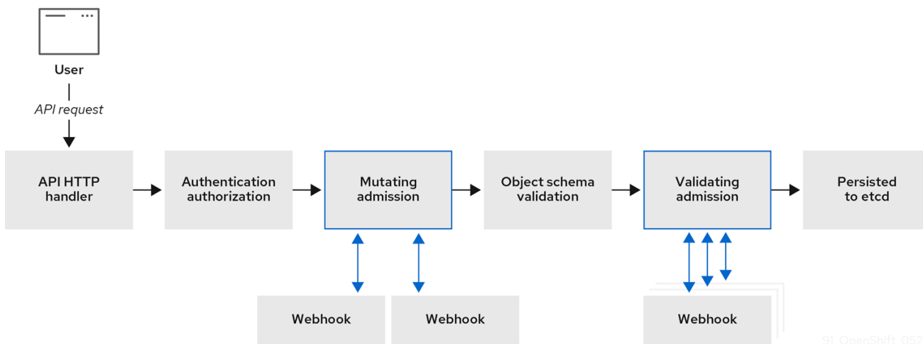
그림 9.1. 변경 및 검증 승인 플러그인을 사용하는 API 승인 체인
