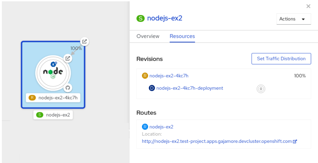
그림 4.1. 서버리스 애플리케이션
