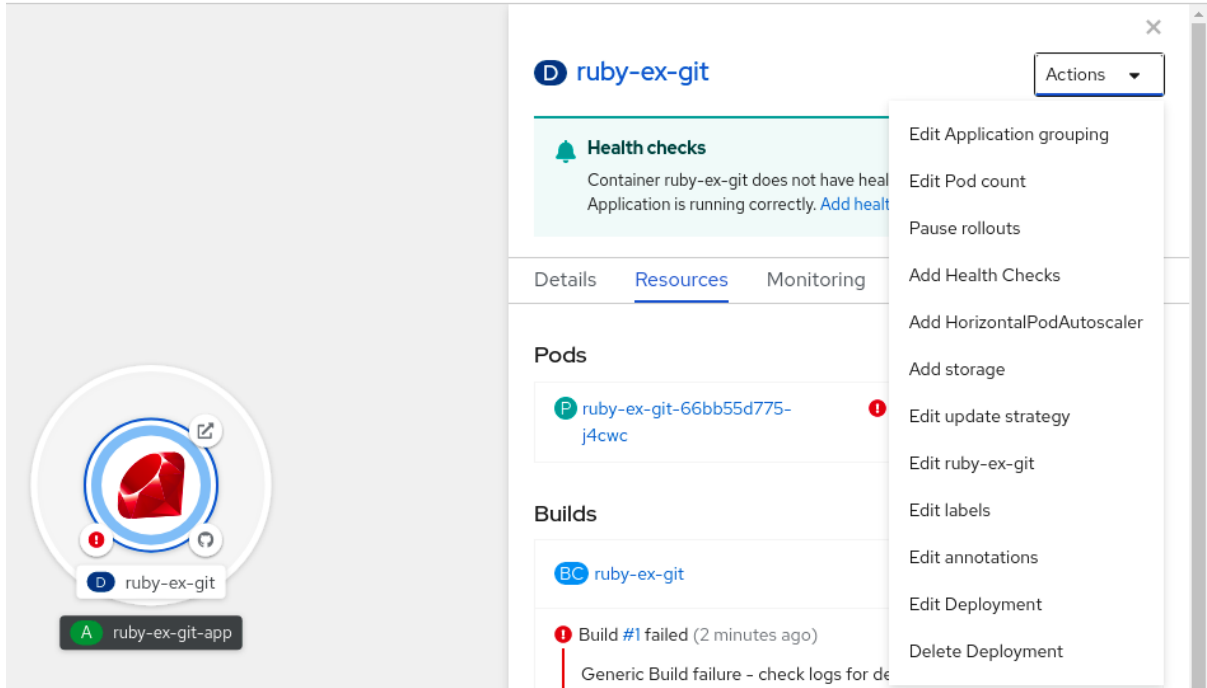
그림 2.2. Add HorizontalPodAutoscaler
