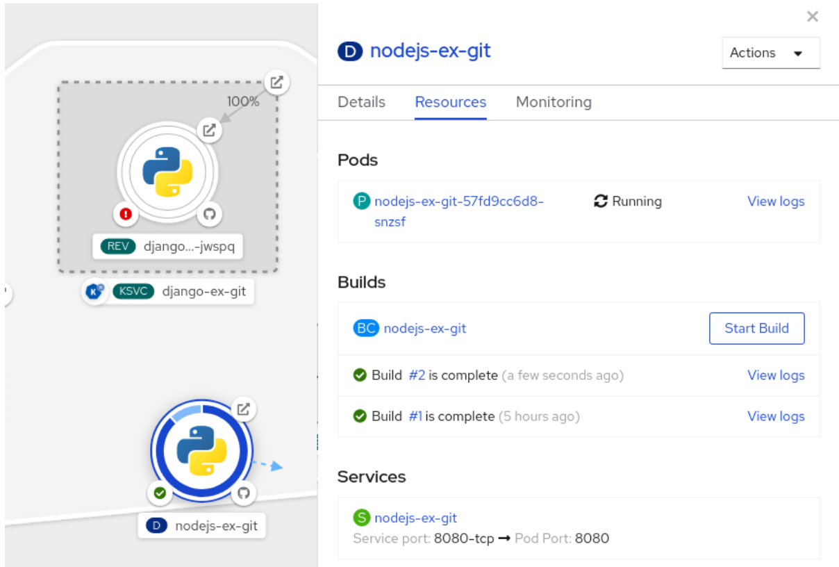
그림 3.12. 애플리케이션 편집 및 재배포
