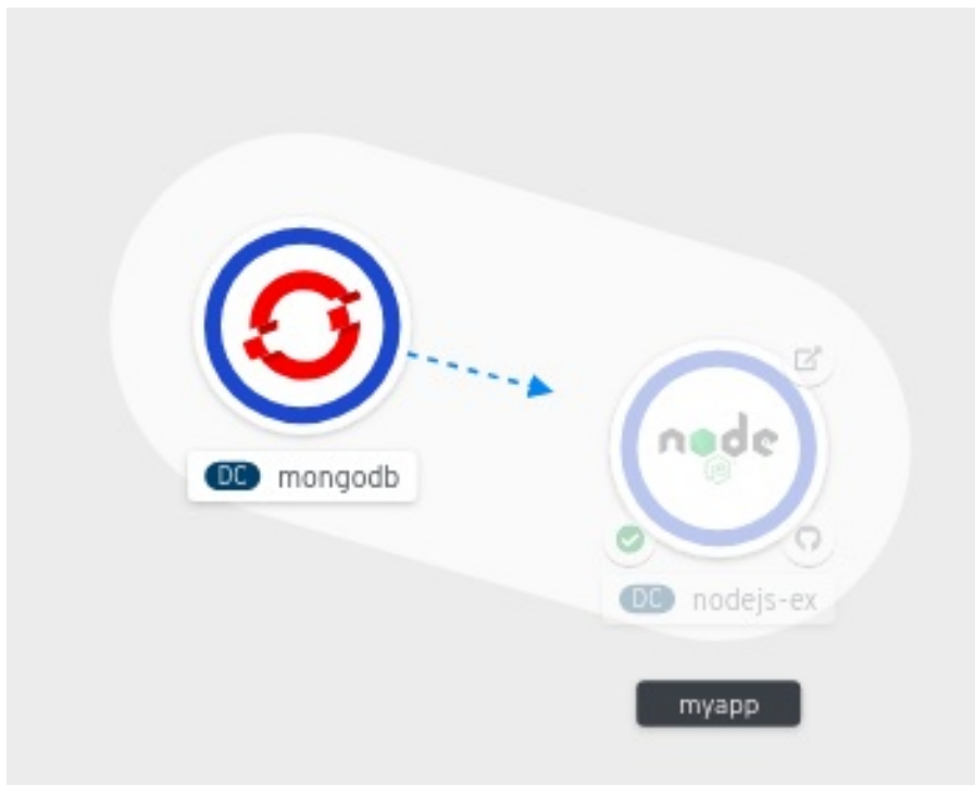
그림 3.7. 커넥터
