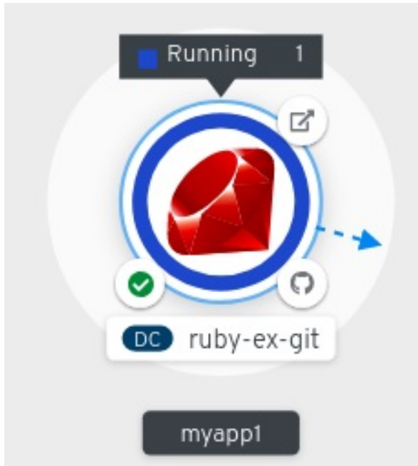
그림 3.3. 애플리케이션 토폴로지
