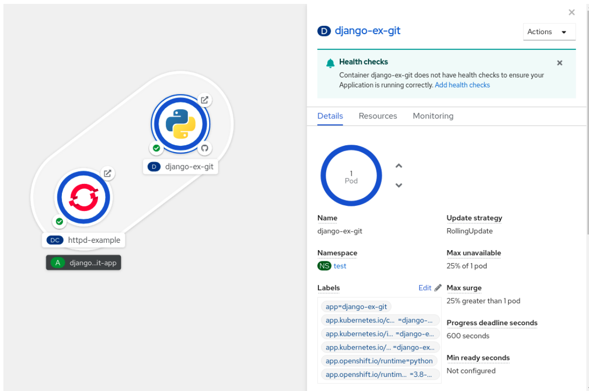
그림 3.6. 애플리케이션 그룹화
