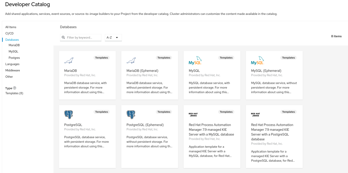
그림 3.1. 개발자 카탈로그
