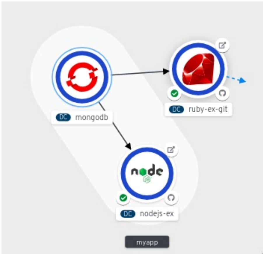
그림 3.8. 여러 애플리케이션 연결
