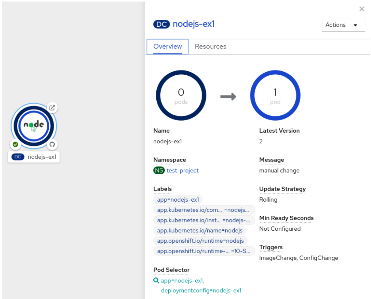
그림 4.1. 롤링 업데이트
