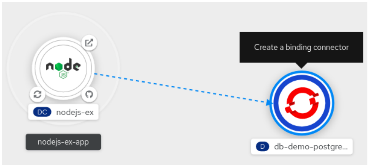
그림 3.9. 바인딩 커넥터
