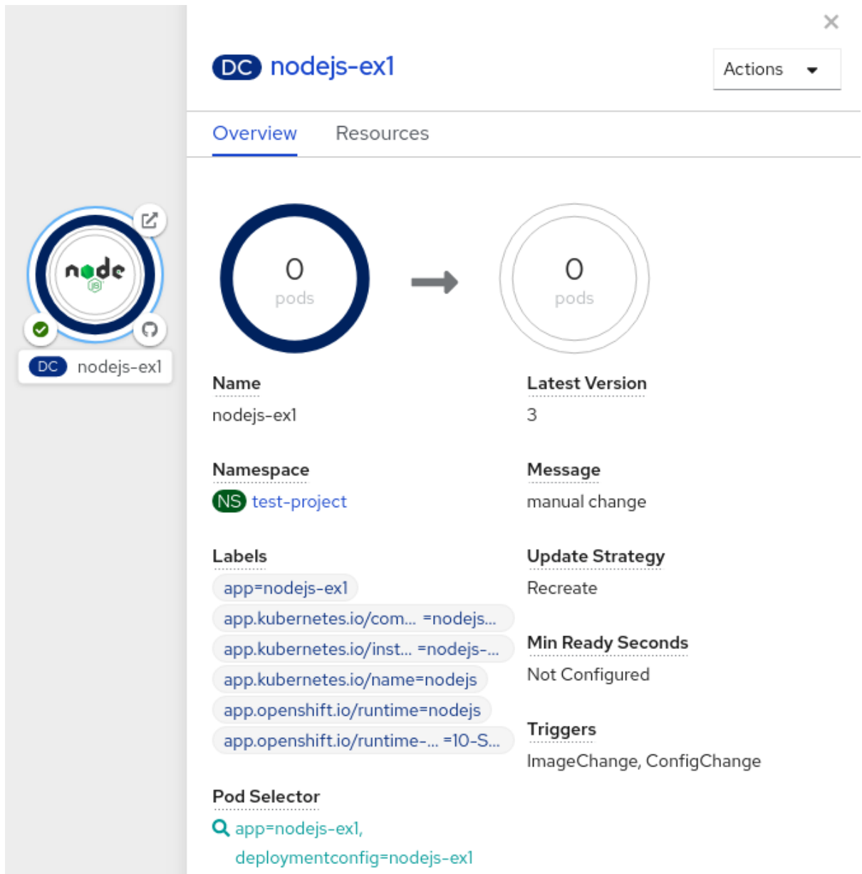
그림 4.2. 재현 업데이트
