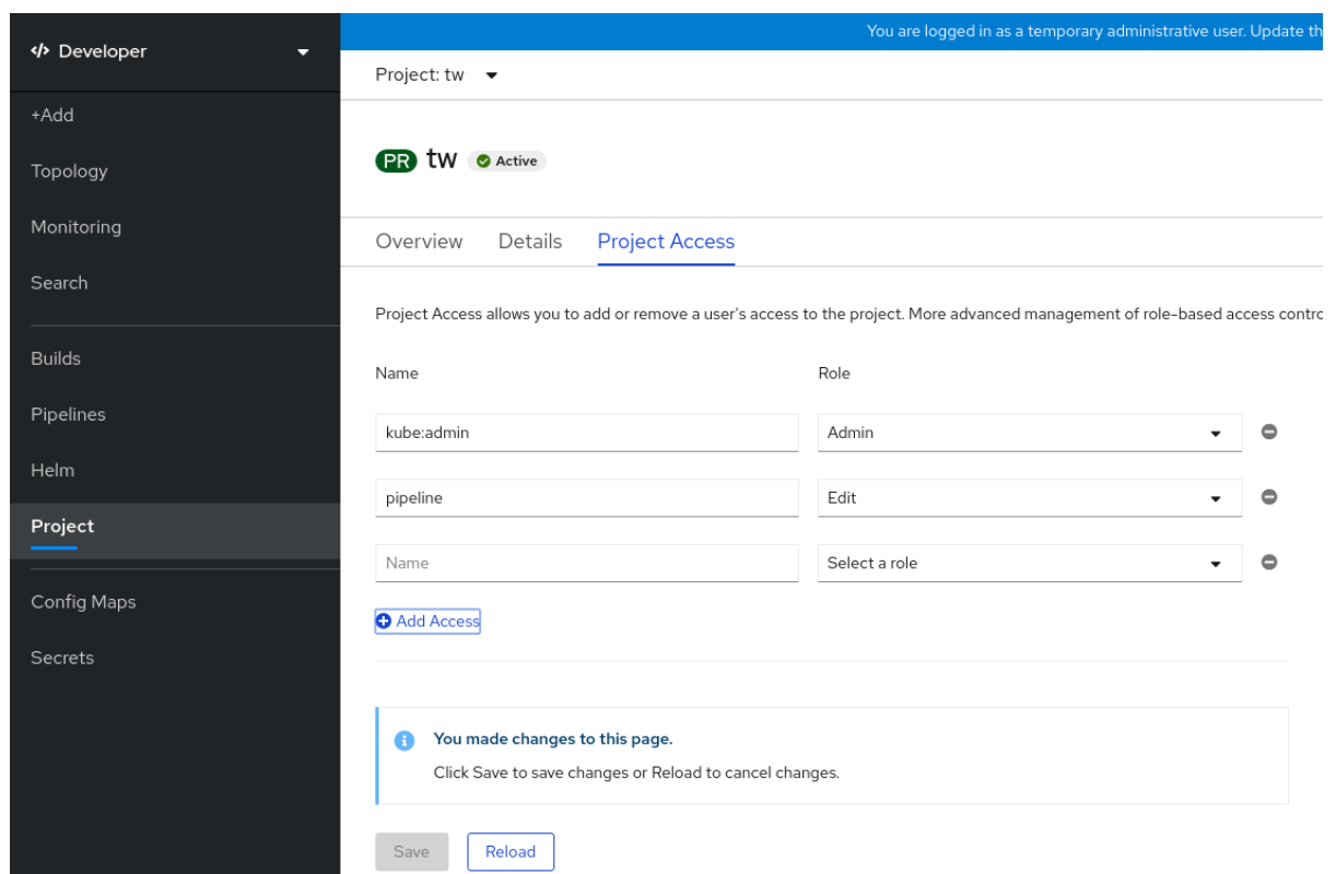
그림 2.2. 프로젝트 권한
