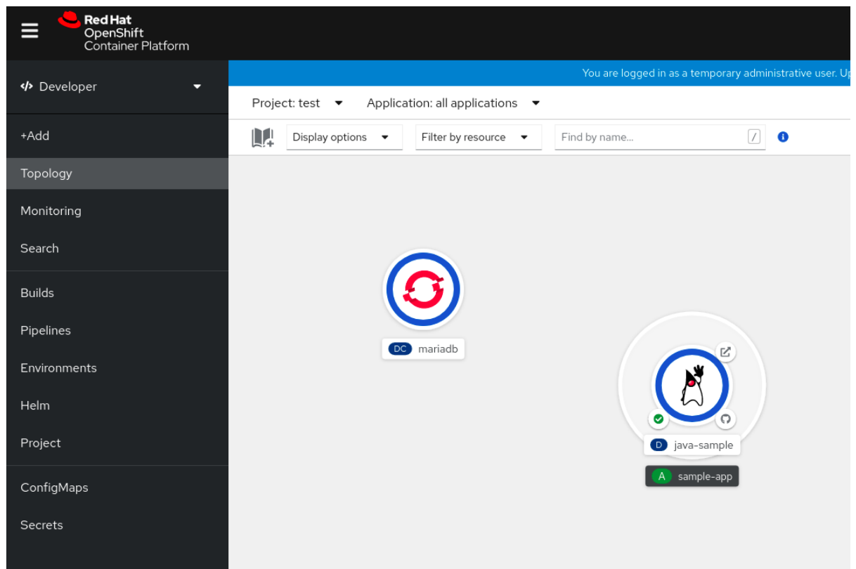
그림 3.2. 토폴로지의 MariaDB
