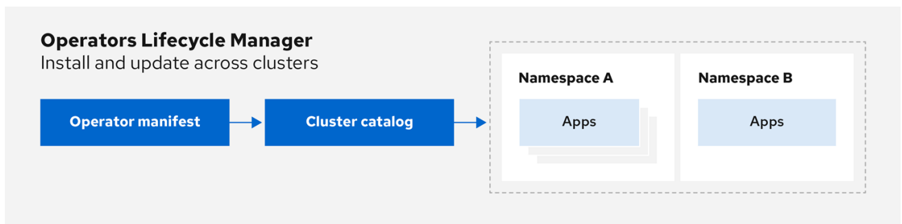
그림 2.2. Operator Lifecycle Manager 워크플로
