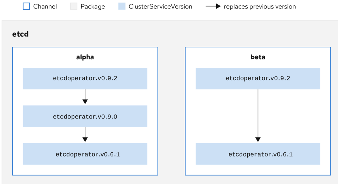
그림 2.4. 카탈로그 소스의 패키지 및 채널
