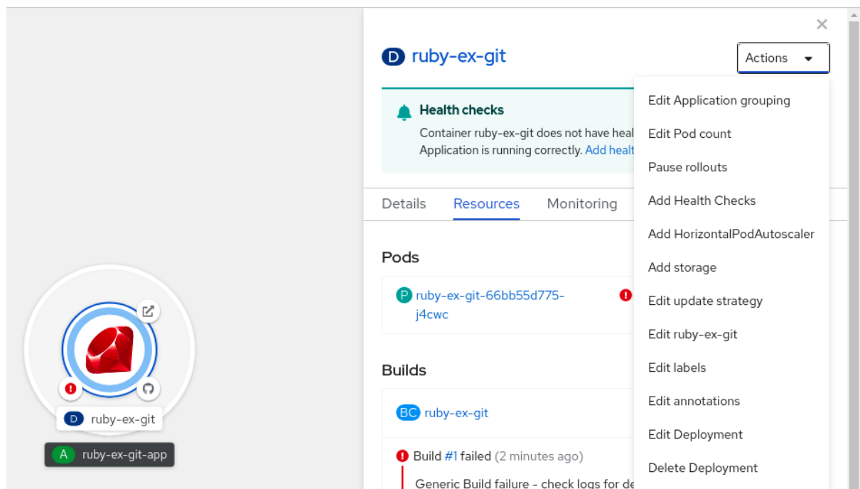
图 2.2. 添加 HorizontalPodAutoscaler
