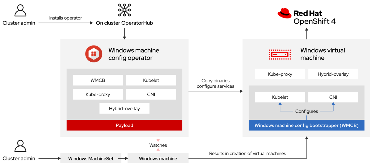
图 3.1. WMCO 设计
