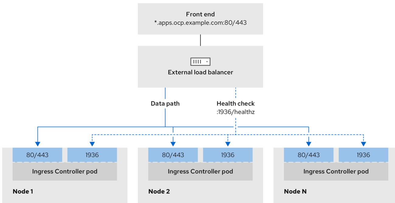
图 14.1. 显示 OpenShift Container Platform 环境中运行的 Ingress Controller 的网络工作流程示例
