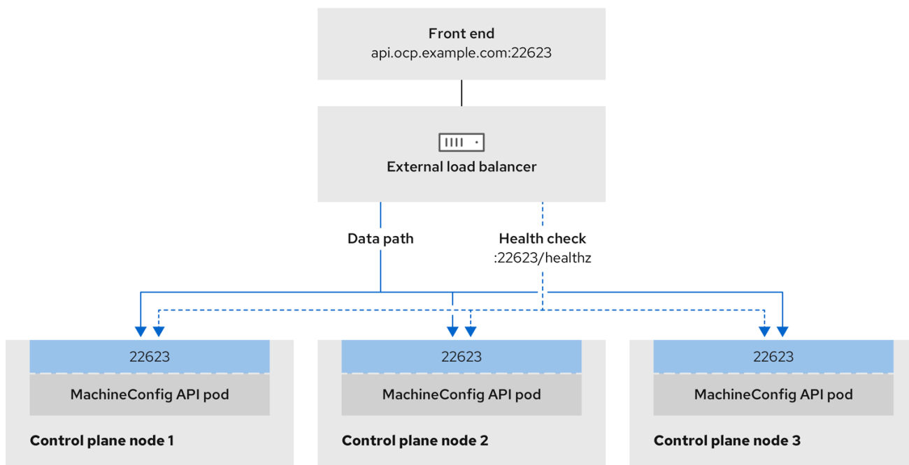
图 22.6. 显示 OpenShift Container Platform 环境中运行的 OpenShift MachineConfig API 的网络工作流程示例
