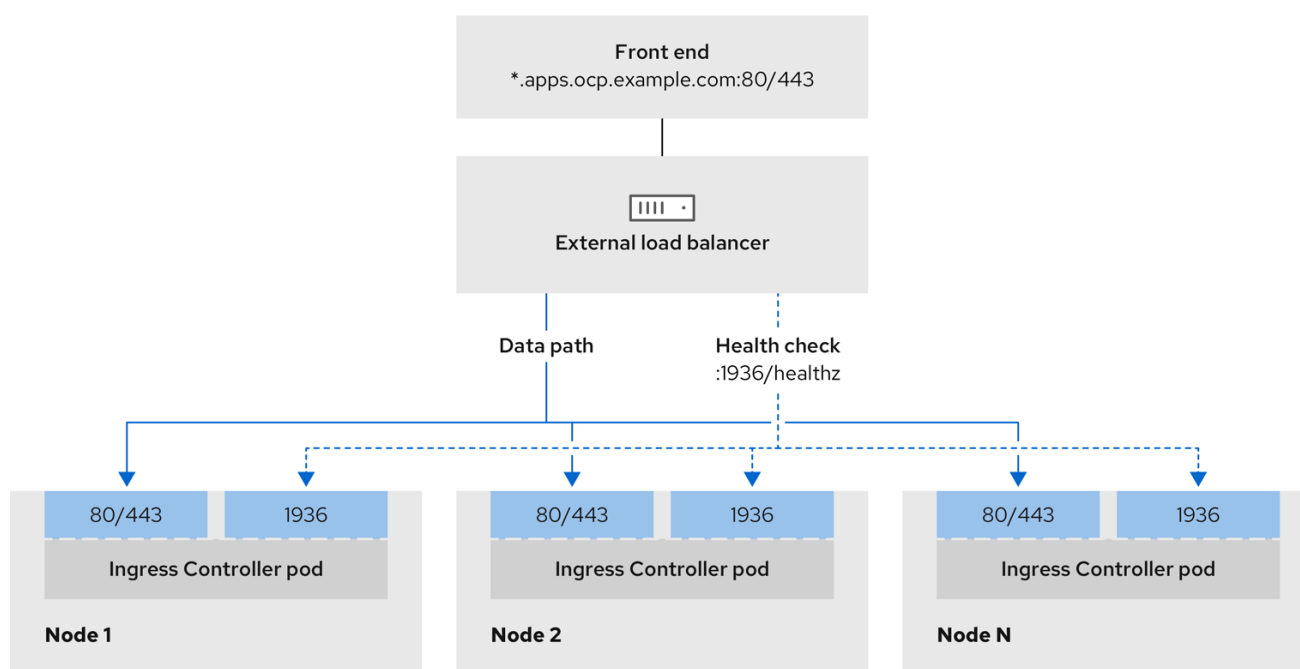
图 21.7. 显示 OpenShift Container Platform 环境中运行的 Ingress Controller 的网络工作流程示例
