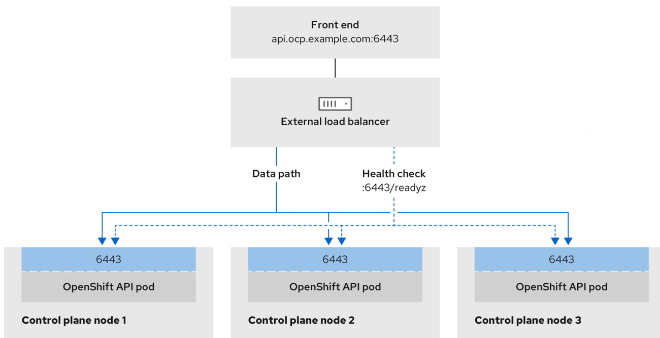
图 22.5. 显示 OpenShift Container Platform 环境中运行的 OpenShift API 的网络工作流示例
