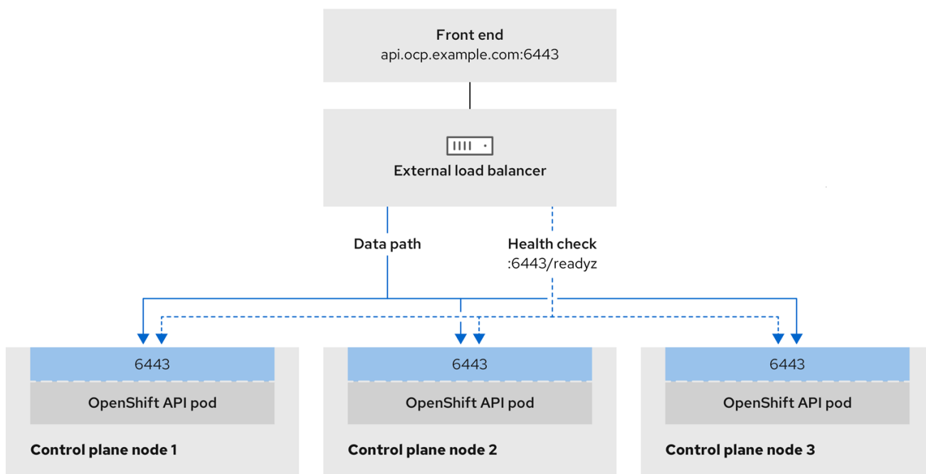
图 22.11. 显示 OpenShift Container Platform 环境中运行的 OpenShift API 的网络工作流程示例
