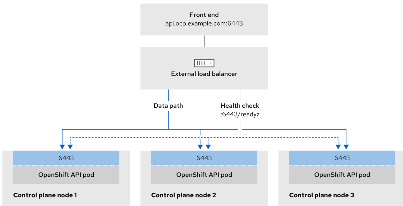
图 21.8. 显示 OpenShift Container Platform 环境中运行的 OpenShift API 的网络工作流程示例
