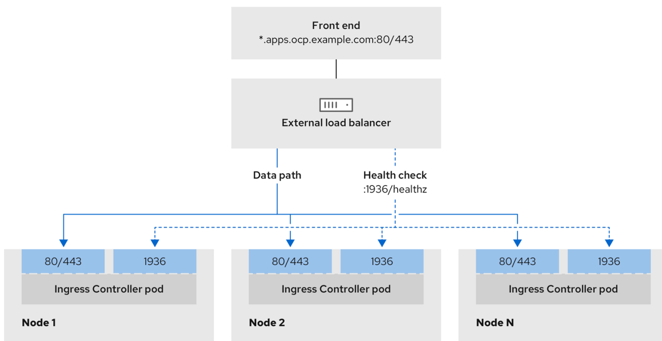
图 22.4. 显示 OpenShift Container Platform 环境中运行的 Ingress Controller 的网络工作流示例
