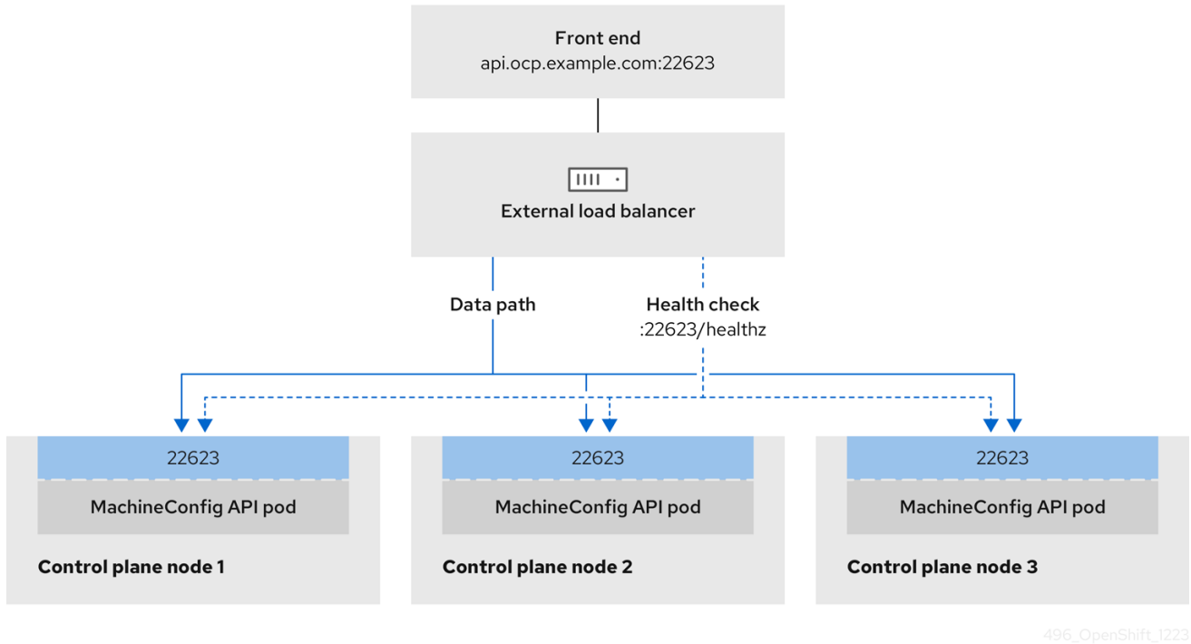
图 22.12. 显示 OpenShift Container Platform 环境中运行的 OpenShift MachineConfig API 的网络工作流示例
