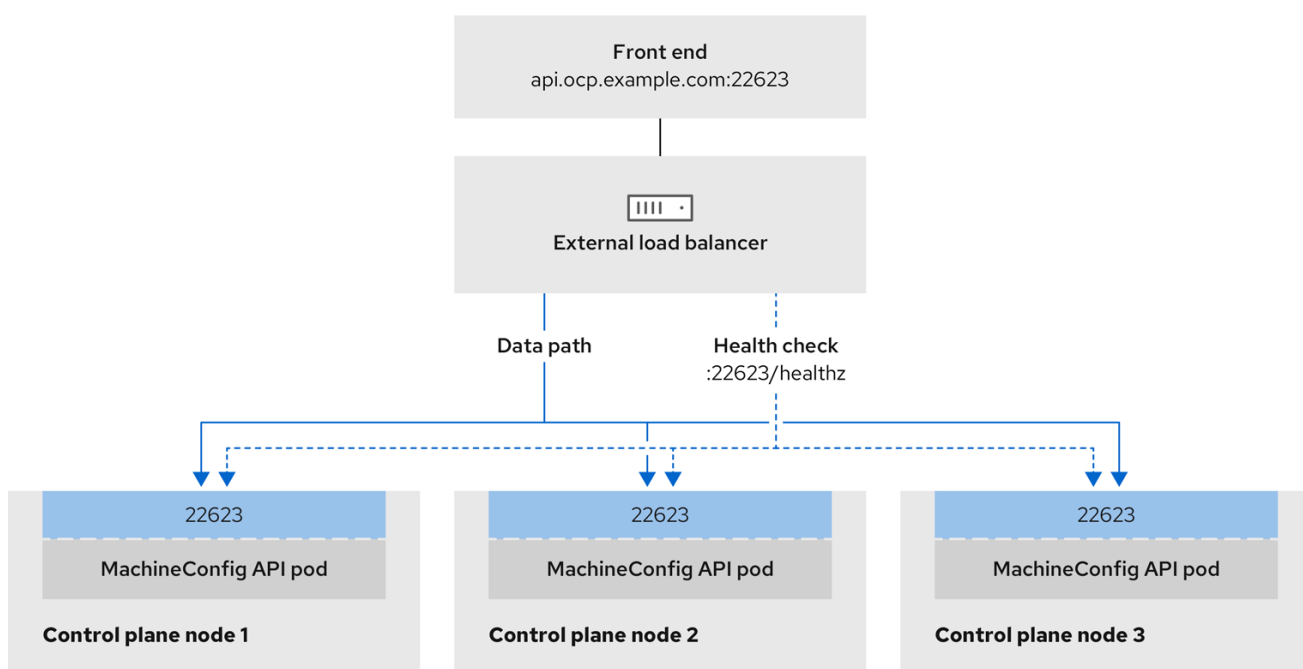
图 21.3. 显示 OpenShift Container Platform 环境中运行的 OpenShift MachineConfig API 的网络工作流程示例
