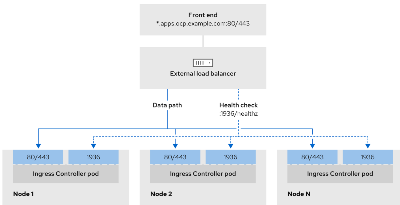
图 22.10. 显示 OpenShift Container Platform 环境中运行的 Ingress Controller 的网络工作流程示例
