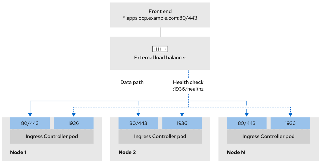
图 21.1. 显示 OpenShift Container Platform 环境中运行的 Ingress Controller 的网络工作流程示例
