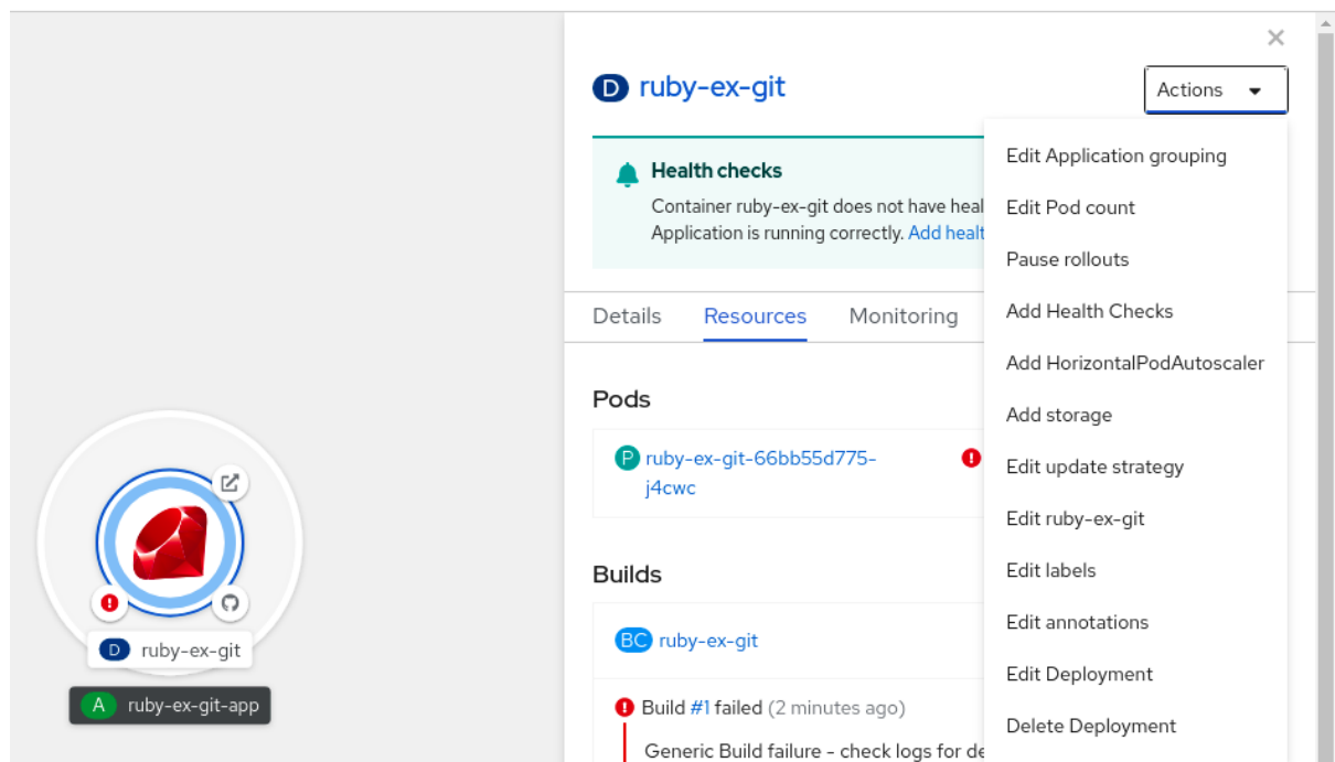
图 2.2. 添加 HorizontalPodAutoscaler
