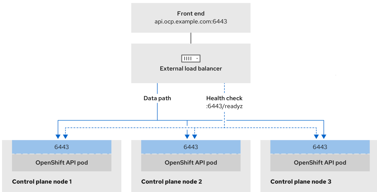
图 24.11. 显示 OpenShift Container Platform 环境中运行的 OpenShift API 的网络工作流程示例
