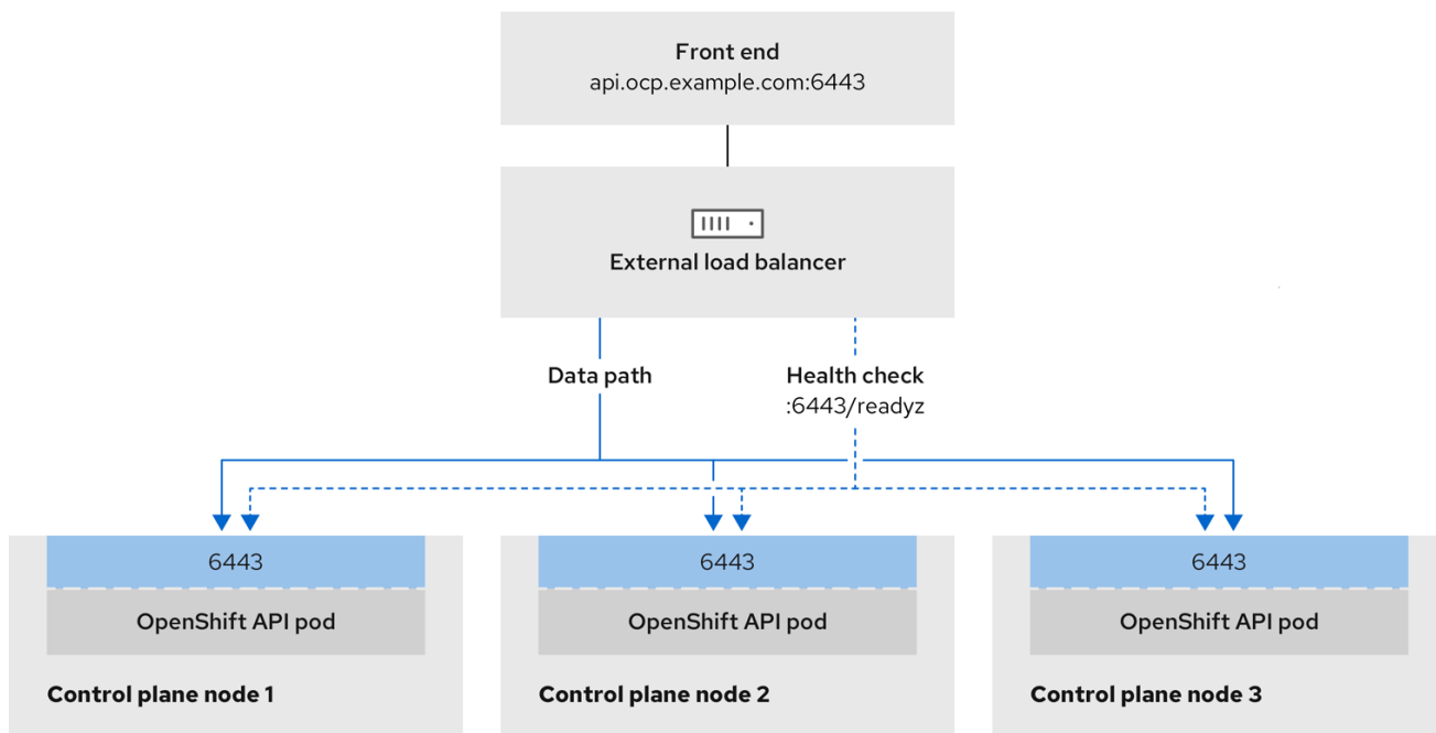
图 24.8. 显示 OpenShift Container Platform 环境中运行的 OpenShift API 的网络工作流示例
