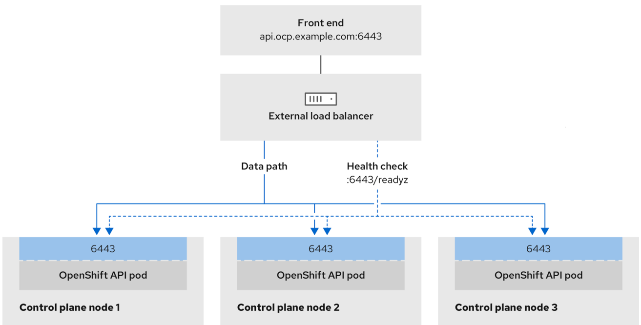
图 23.8. 显示 OpenShift Container Platform 环境中运行的 OpenShift API 的网络工作流程示例
