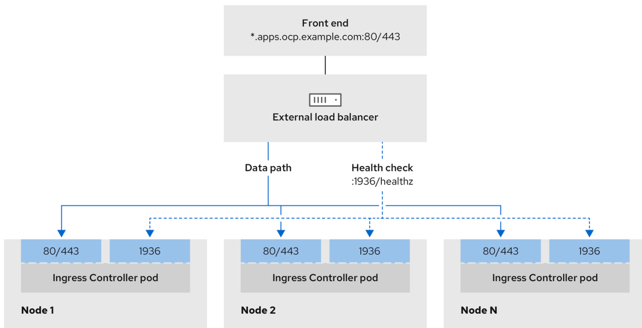
图 24.7. 显示 OpenShift Container Platform 环境中运行的 Ingress Controller 的网络工作流示例
