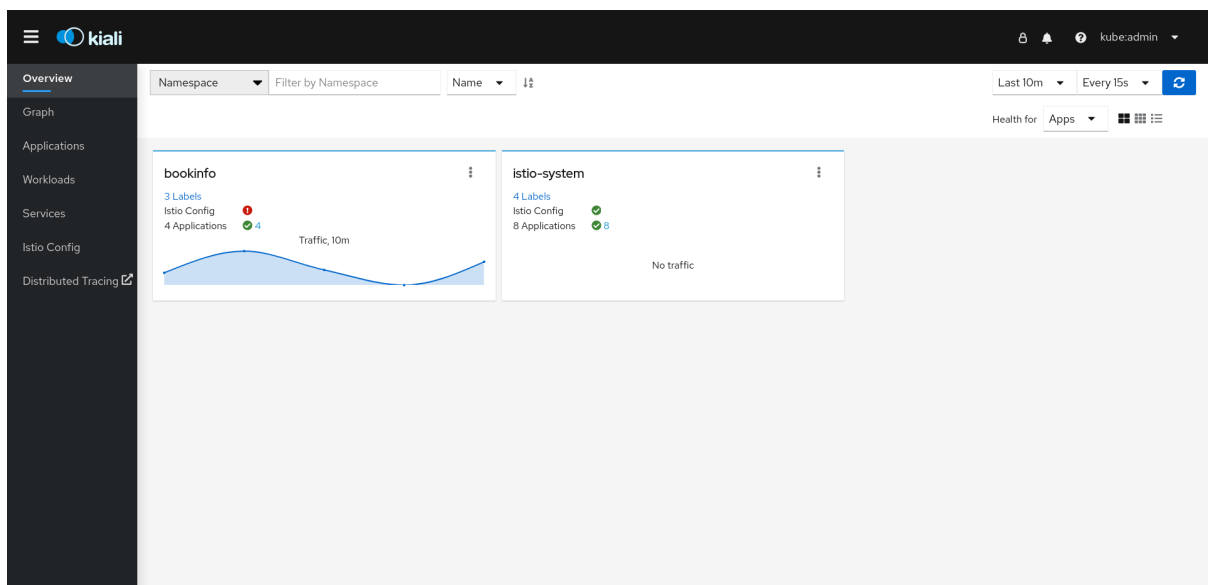
图 1.1. Kiali Overview 页
