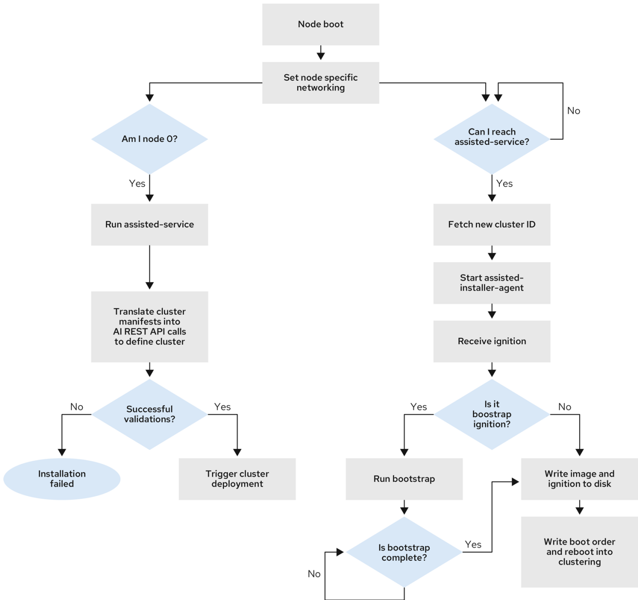
图 14.1. 节点安装 workflow
