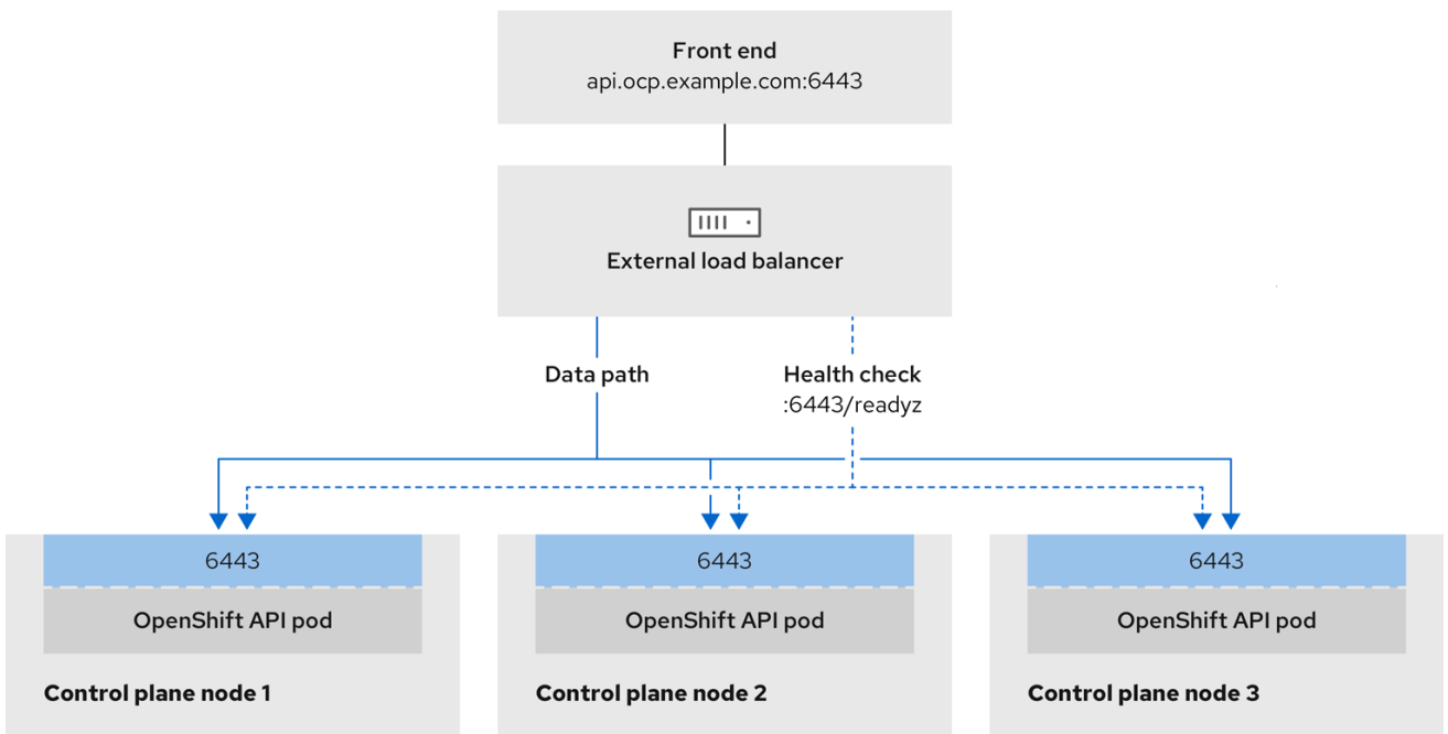
图 24.5. 显示 OpenShift Container Platform 环境中运行的 OpenShift API 的网络工作流程示例
