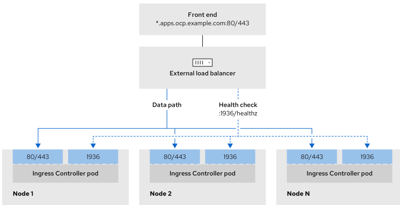
图 24.1. 显示 OpenShift Container Platform 环境中运行的 Ingress Controller 的网络工作流程示例
