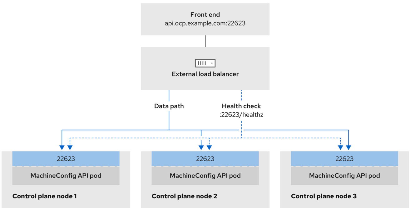
图 21.9. 显示 OpenShift Container Platform 环境中运行的 OpenShift MachineConfig API 的网络工作流程示例
