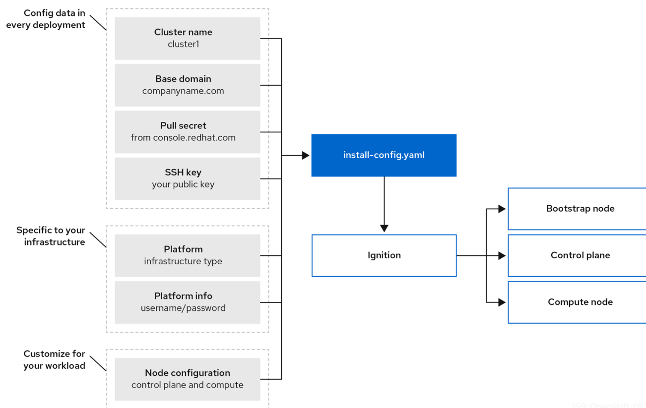
图 1.1. OpenShift Container Platform 安装目标和依赖项
