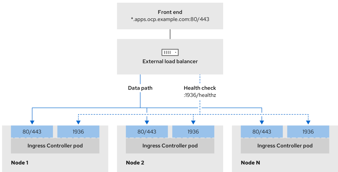
图 21.7. 显示 OpenShift Container Platform 环境中运行的 Ingress Controller 的网络工作流程示例
