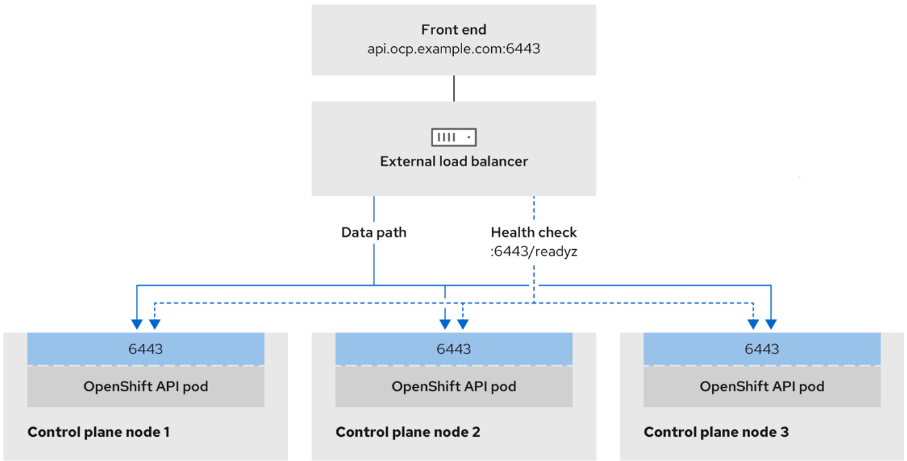
图 21.8. 显示 OpenShift Container Platform 环境中运行的 OpenShift API 的网络工作流程示例
