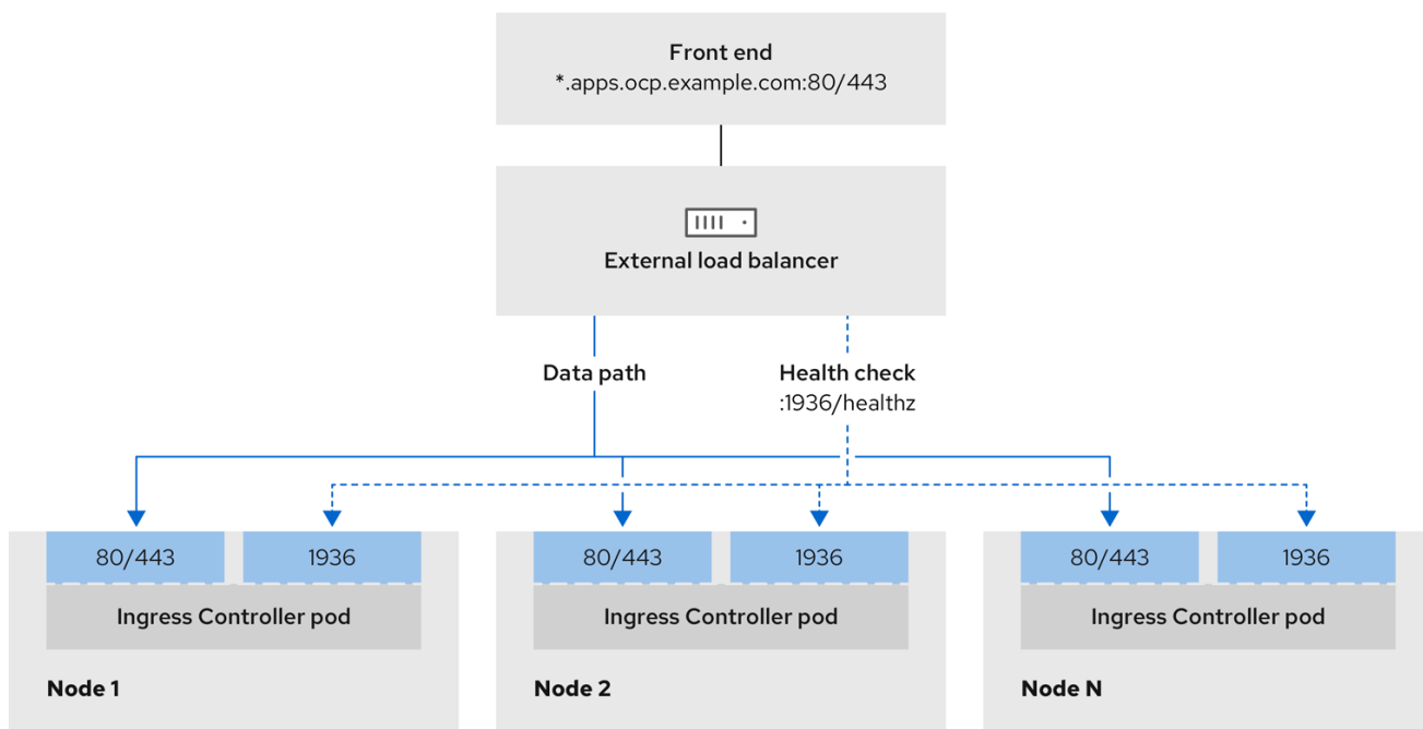
图 21.1. 显示 OpenShift Container Platform 环境中运行的 Ingress Controller 的网络工作流程示例
