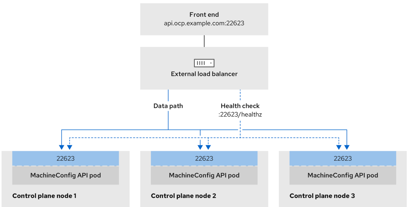
图 21.6. 显示 OpenShift Container Platform 环境中运行的 OpenShift MachineConfig API 的网络工作流程示例
