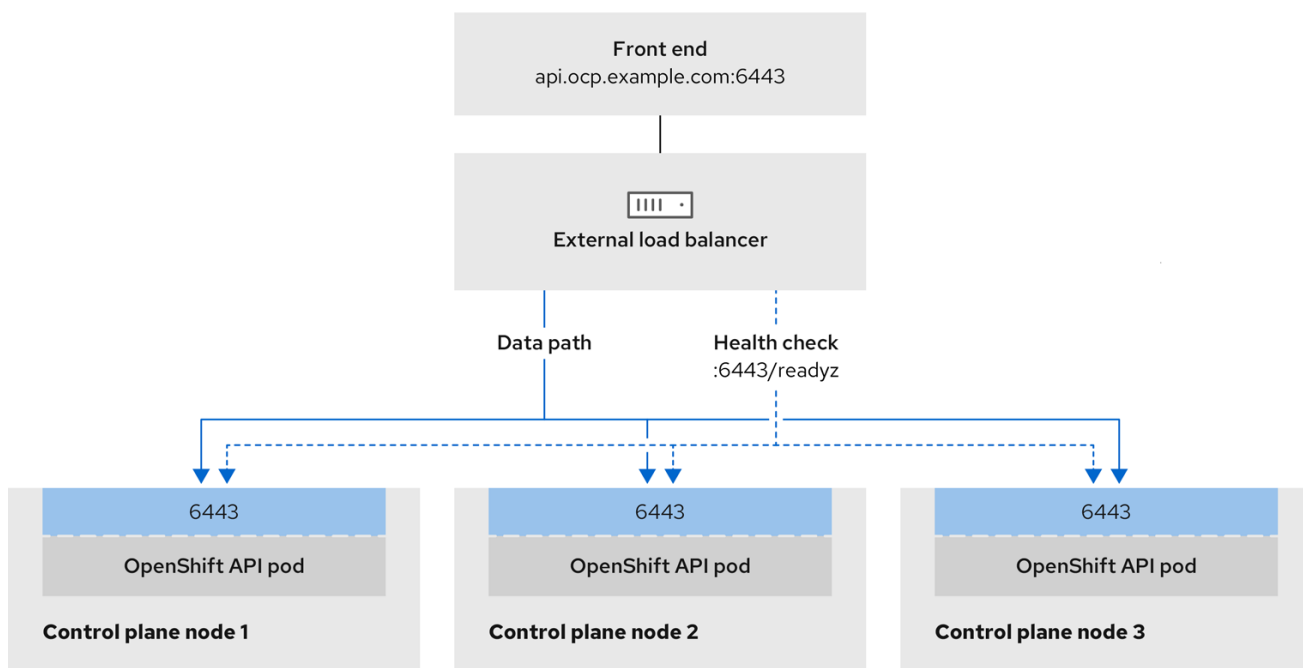
图 21.2. 显示 OpenShift Container Platform 环境中运行的 OpenShift API 的网络工作流程示例
