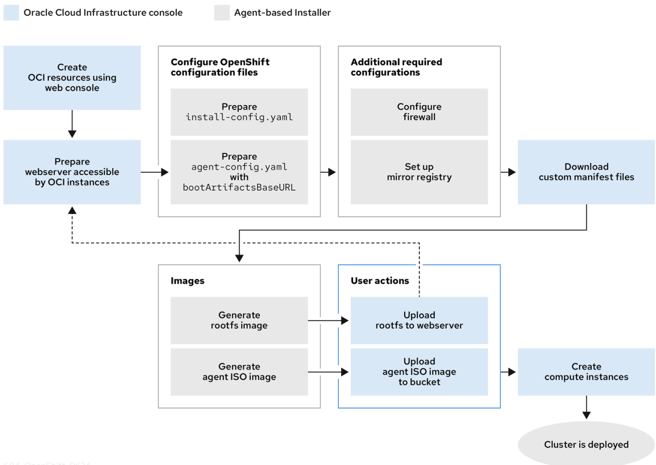
图 20.4. 在断开连接的环境中使用基于代理的安装程序在 OCI 上安装集群的工作流
