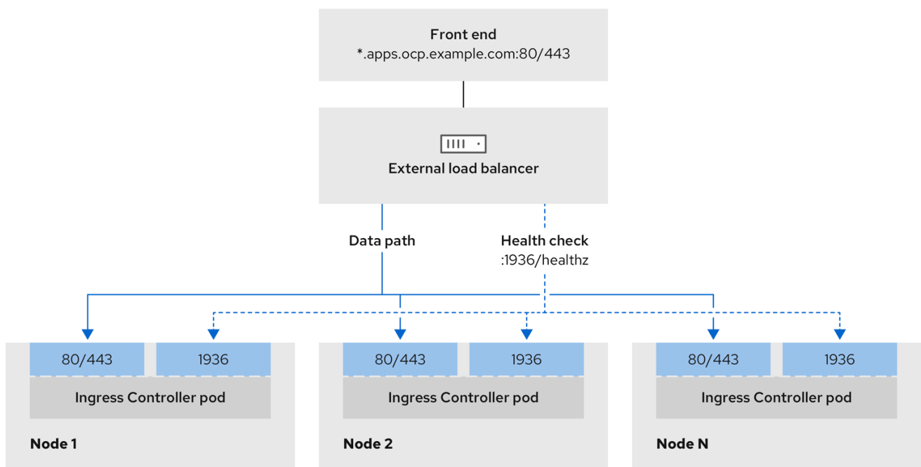
图 21.4. 显示 OpenShift Container Platform 环境中运行的 Ingress Controller 的网络工作流程示例
