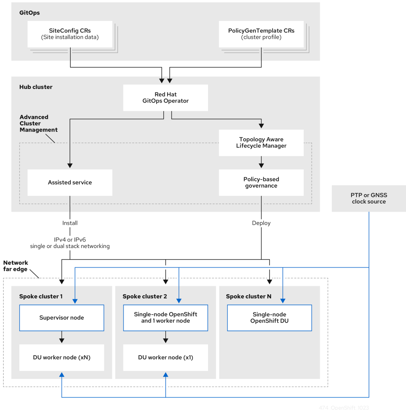
图 2.1. Telco RAN DU 部署架构概述
