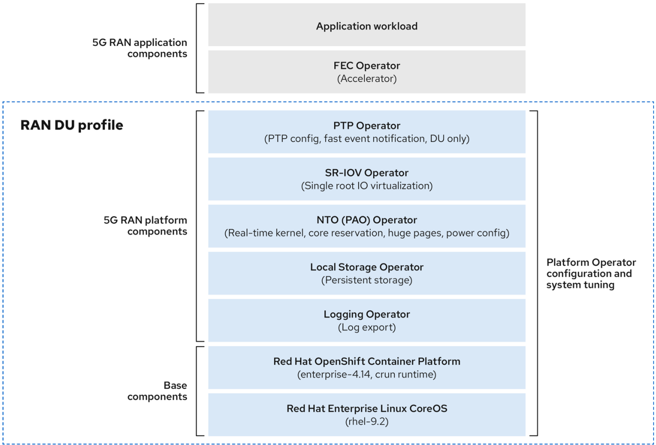
图 2.2. Telco RAN DU 参考组件
