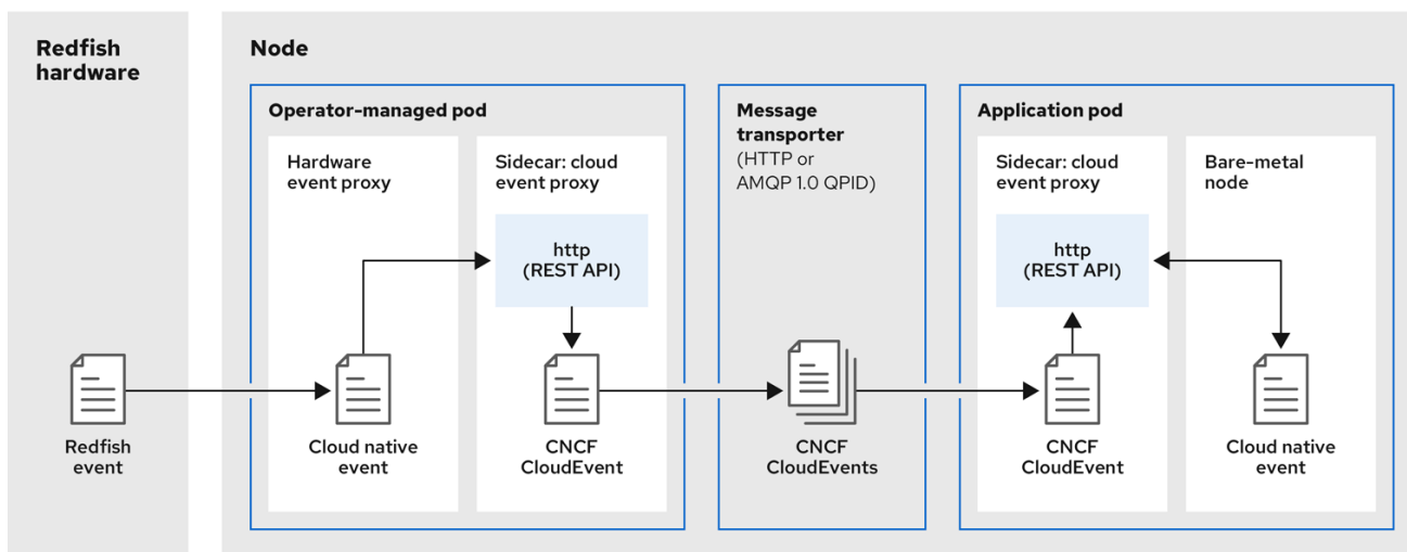
图 10.1. 裸机事件中继数据流
