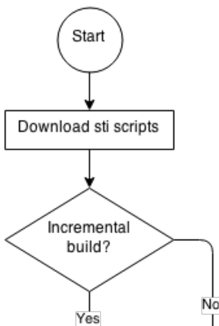
图 5.1. 构建工作流
