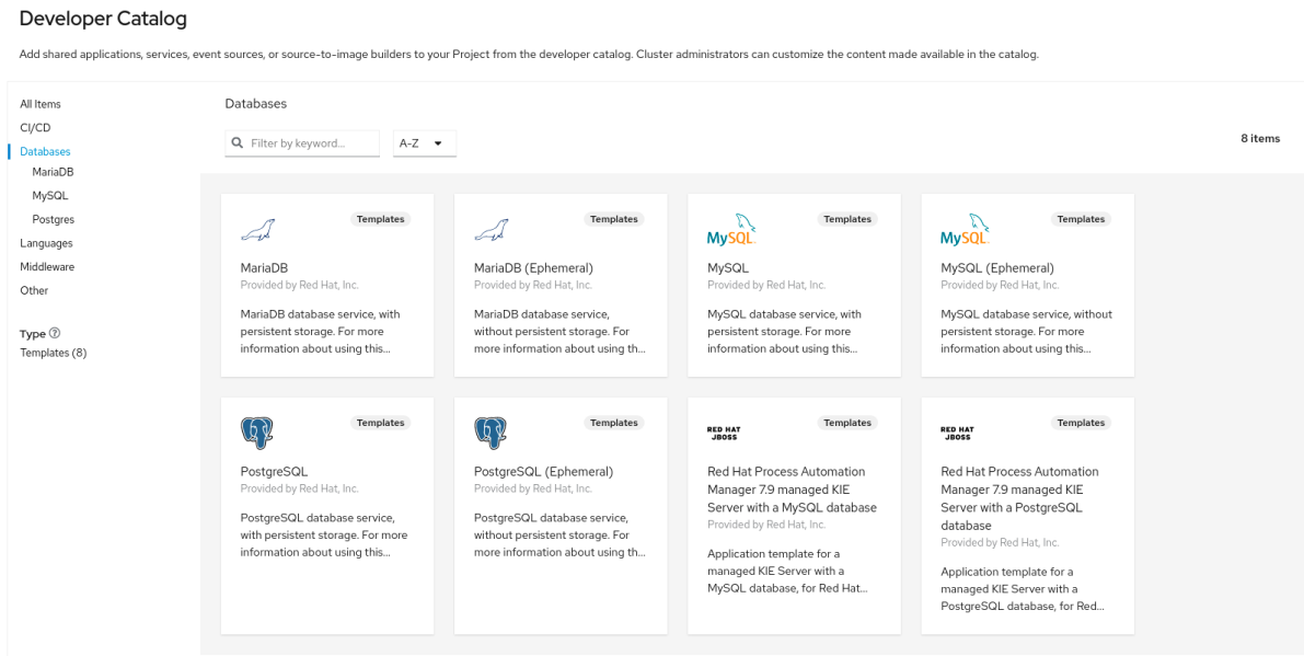
图 3.1. 开发者目录
