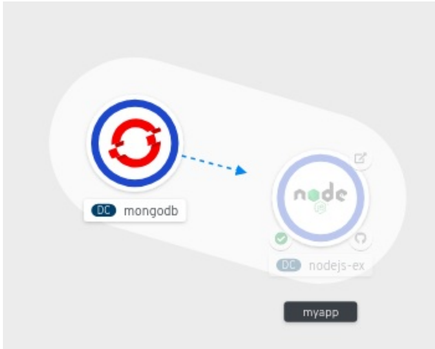
图 3.7. 连接器
