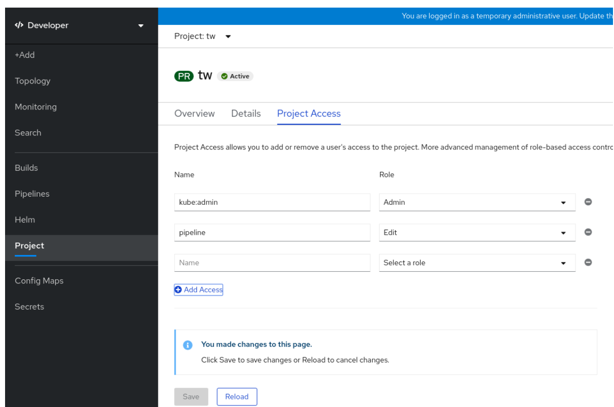
图 2.2. 项目权限
