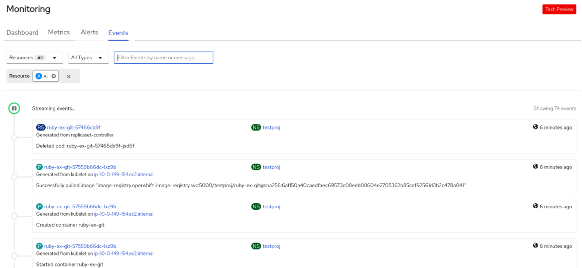
图 7.4. 监控事件
