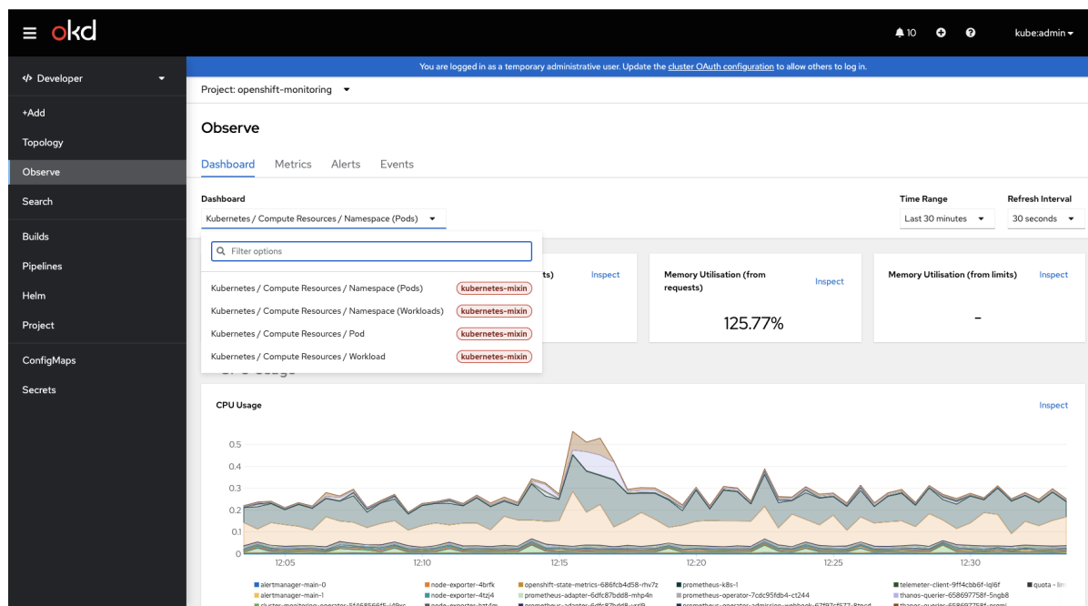
图 9.1. 观察仪表板
