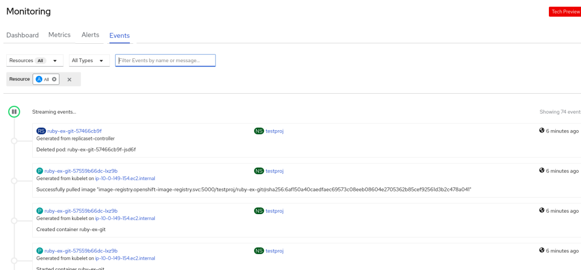
图 9.4. 监控事件
