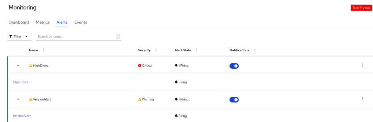
图 9.3. 监控警报
