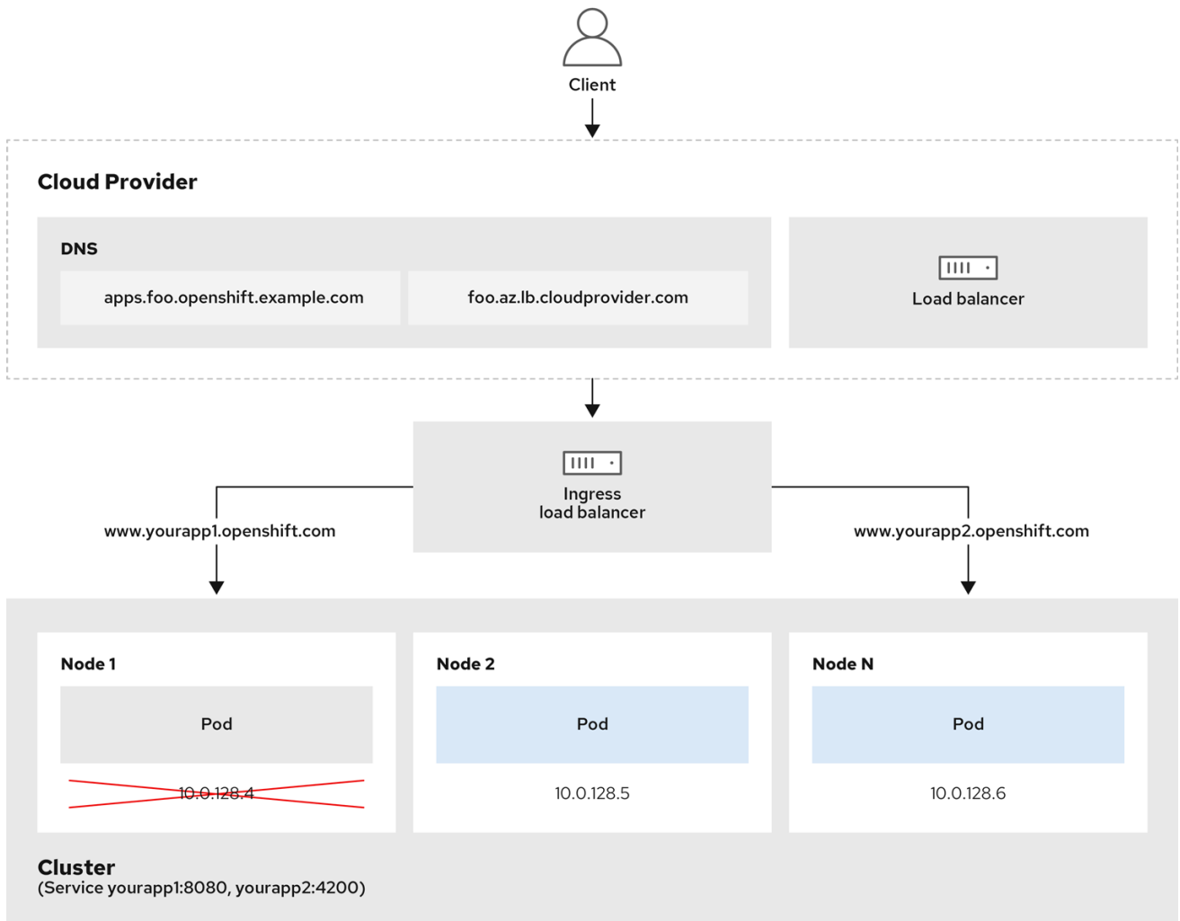
图 2.1. LoadBalancer 图表
