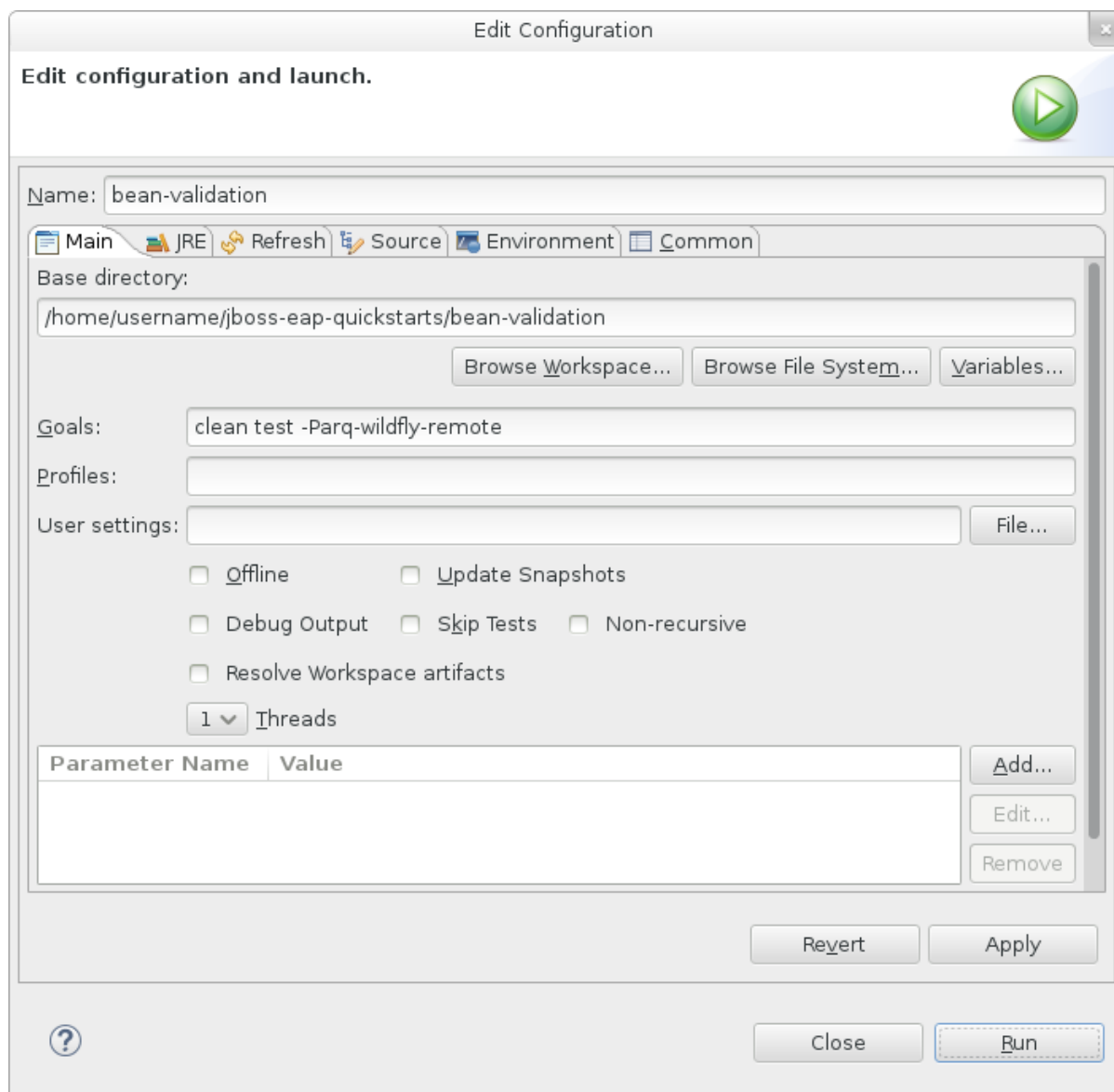
图 3.12. 编辑配置
