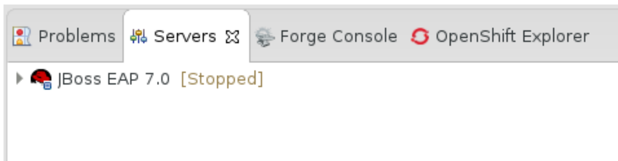
图 3.6. 服务器列表
