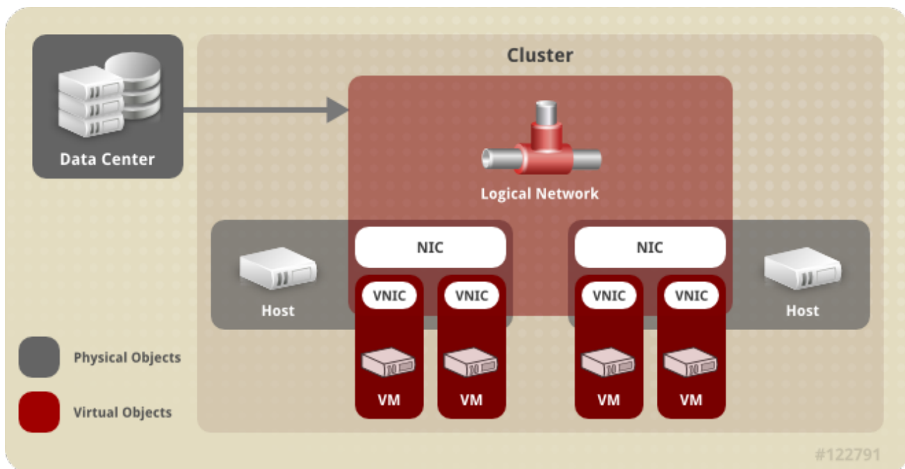
图 1.3. 网络架构
