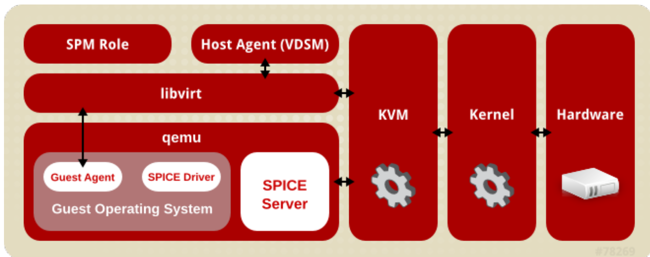
图 1.2. 主机的构架
