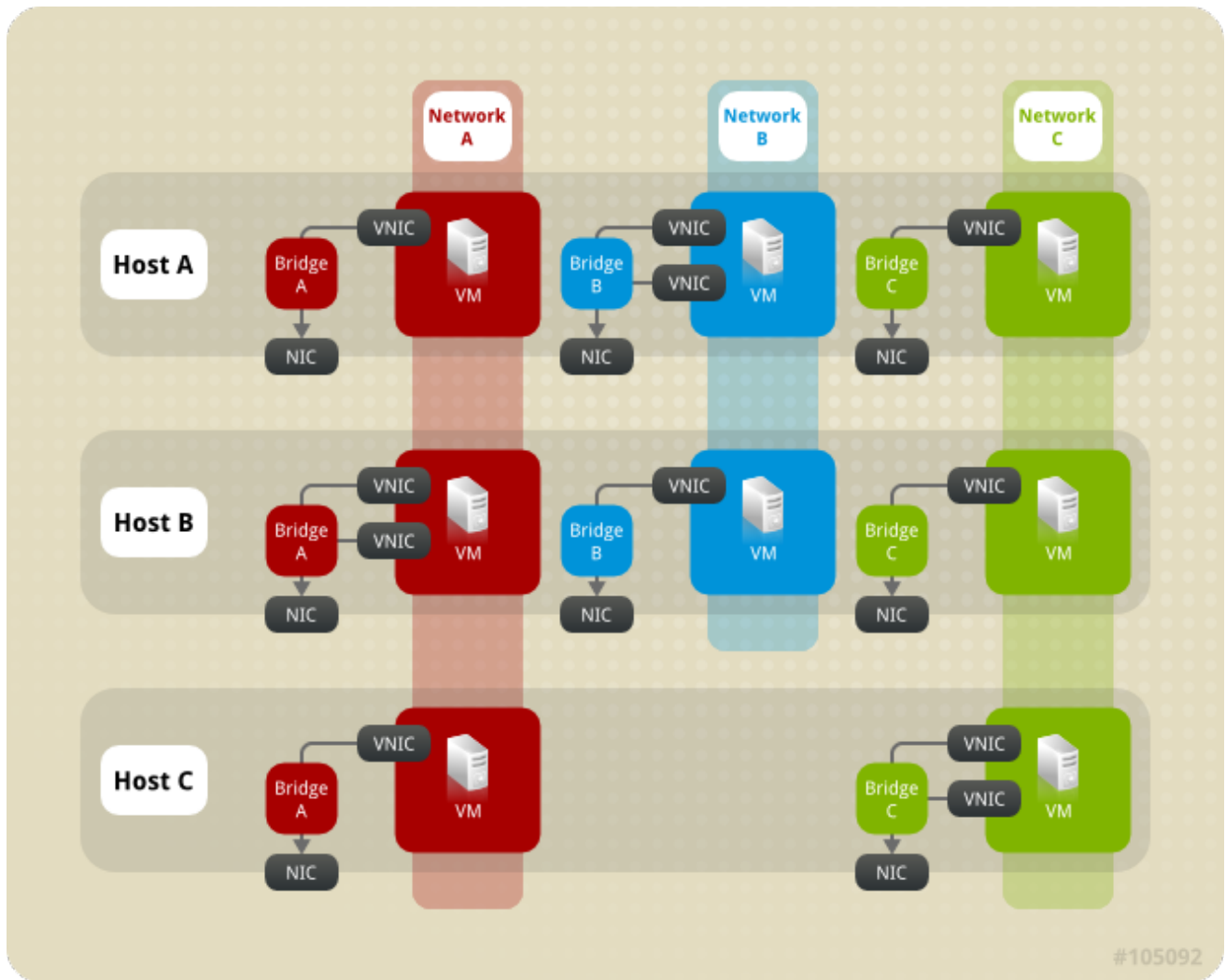
图 3.1. 一个集群内的网络
