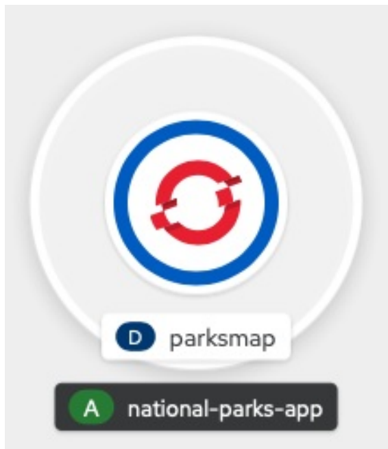
图 3.2. Parksmap 部署
